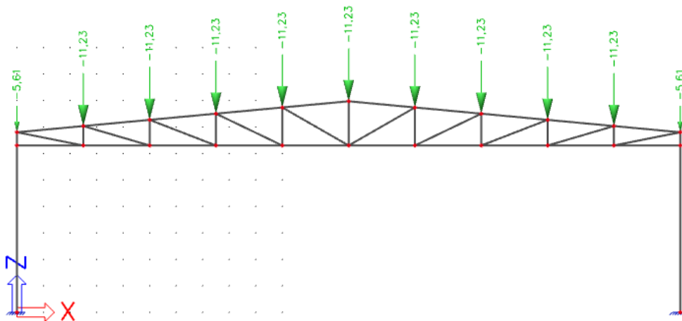
Slika 2.3. Promjenjivo opterećenje
