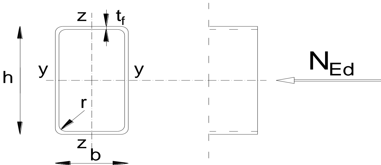
Slika 40 Poprečni presjek vertikalna
