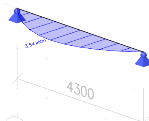
Slika 30 Dijagram momenata M_y i M_z za kombinaciju 3
