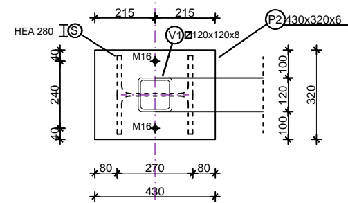
Presjek 2-2
