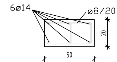
Presjek 2-2 MJ 1:25
