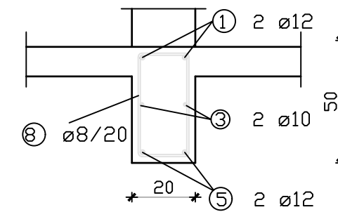
Presjek 1-1 MJ 1:25
