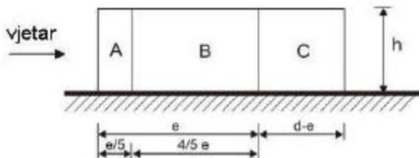
Slika 11. Prikaz područja vjetra za vertikalne zidove - bočni pogled
