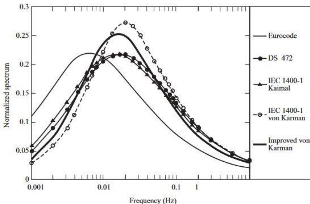
Slika 8-1 Usporedba spektara na glatkom terenu pri 10 m/s [12]
