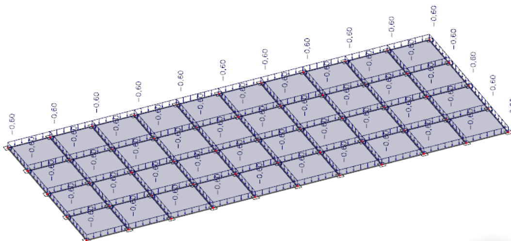
Slika 4.2 Korisno opterećenje
