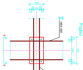
DETALJ "H" SPOJ BOČNE PODROŽNICE NA STUP
