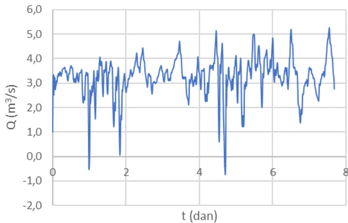
Slika 51. Hidrogram 16. elementa
