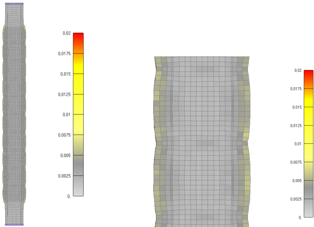
Slika 6.25: Prikaz pukotina za cijeli stup nakon 30 minuta (lijevo-cijeli stup, desno-detalj stupa)
