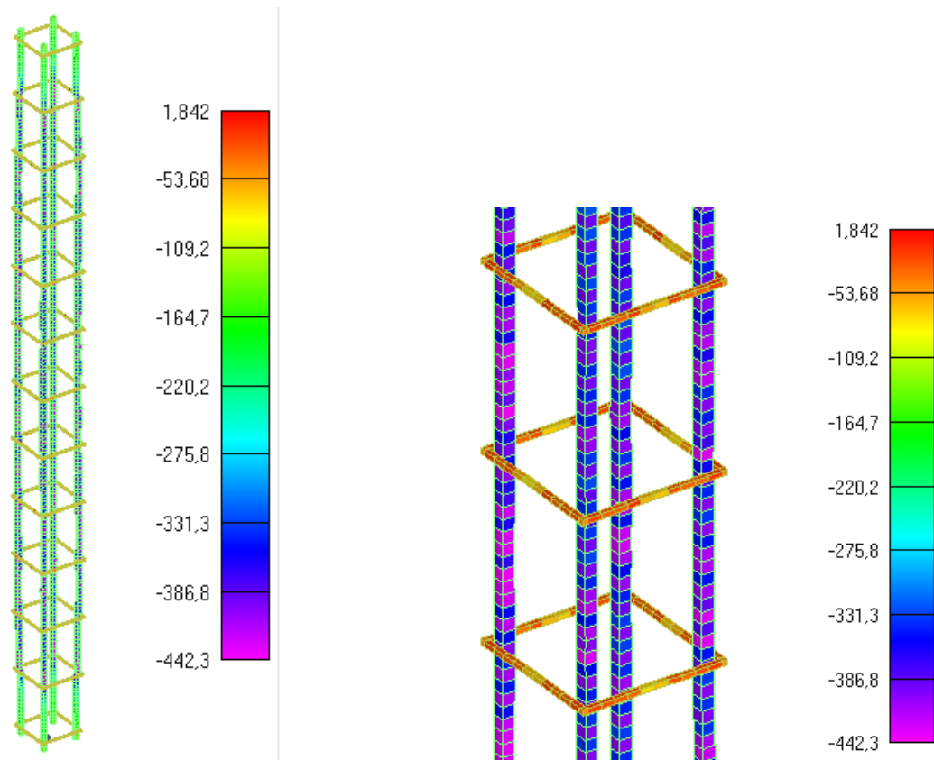
Slika 6.37: Prikaz napreznja glavne uzdužne armature i spona za djelovanje požara od 90min (lijevo-cijeli stup, desno-detalj stupa)
