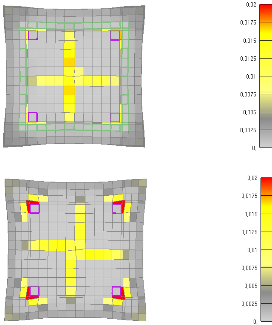
Slika 6.80: Prikaz pukotina za poprečni presjek stupa nakon 30 minuta požara (gore-sa sponama, dolje-bez spona)
