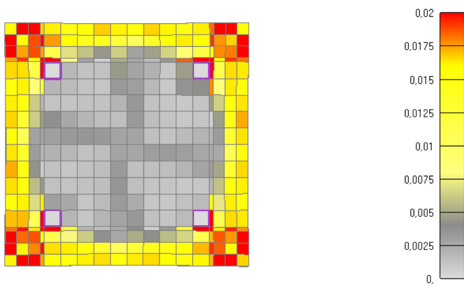
Slika 6.144: Prikaz pukotina za poprečni presjek stupa nakon 1030 minuta (gore-sa sponama, dolje-bez spona)
