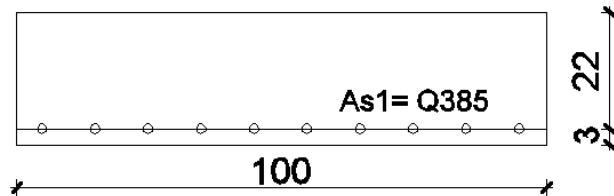
Slika 4.22. Skica armature ploče u polju
