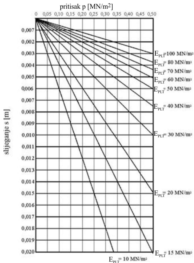
Slika 5.10 Obrazac za određivanje modula stišljivosti na terenu
