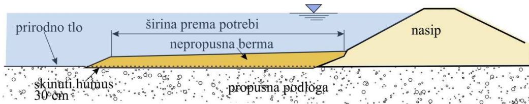
Slika 9.32 Uzvodna berma
