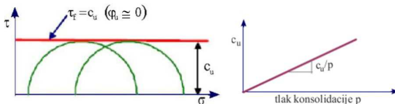
Slika 4.10 Troosni nekonsolidirani, nedrenirani pokus potpuno zasićenog tla i ovisnost nedrenirane kohezije o prethodnoj konsolidaciji
