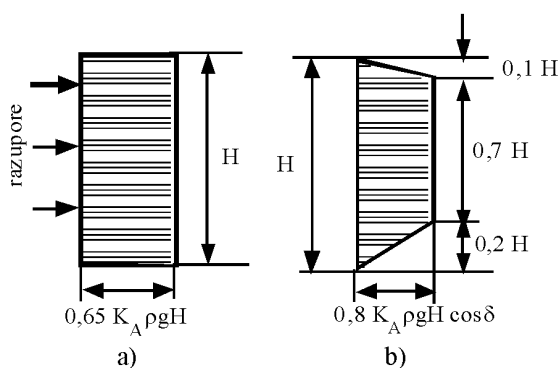
Slika 5.4 Raspodjela pritisaka na podgradu u pijescima (Dismuke, 1991.)
