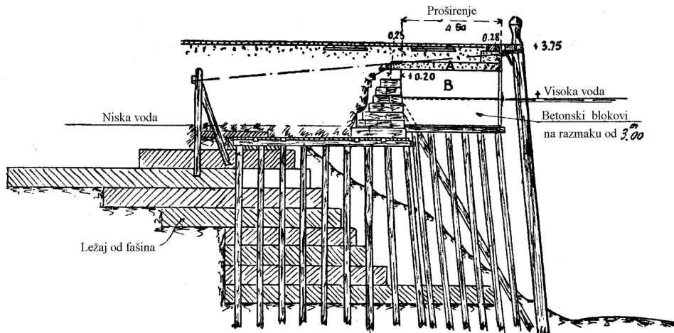
Slika 0.2 Obalni zid u Rotterdamu (Proudon, 1936.)
