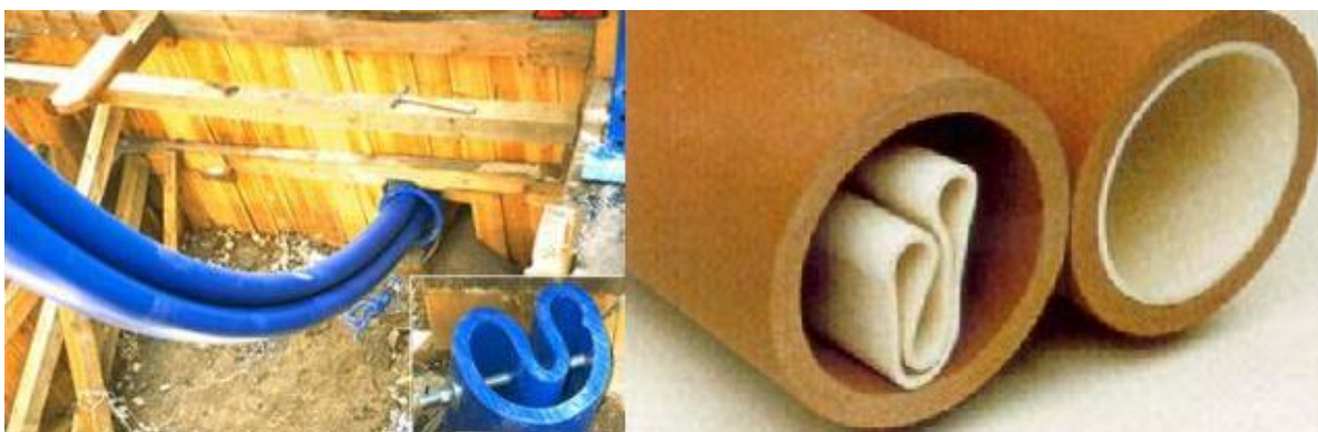
Slika 29. Close-fit lining (Deformed pipe) metoda s presavijanjem cijevi [18]
