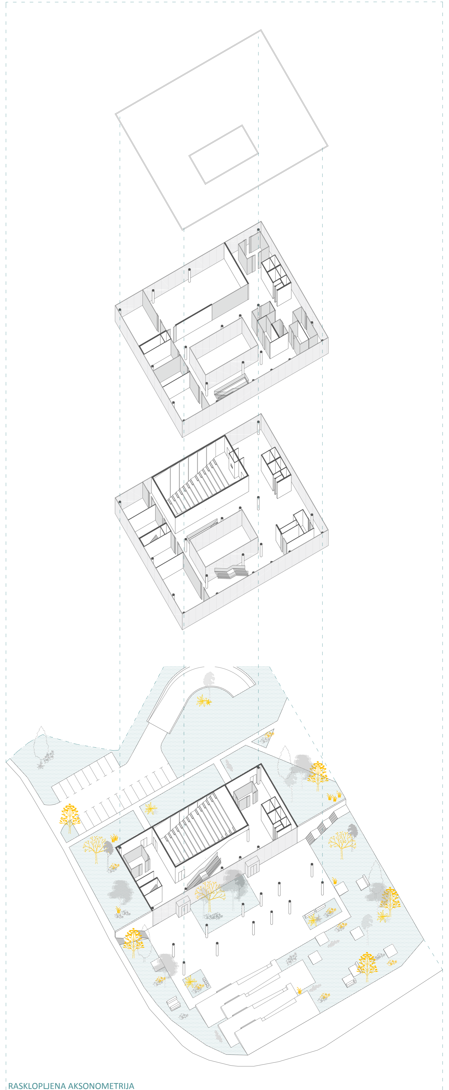
RASKLOPLJENA AKSONOMETRIJA
