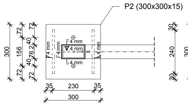
Presjek 2-2
