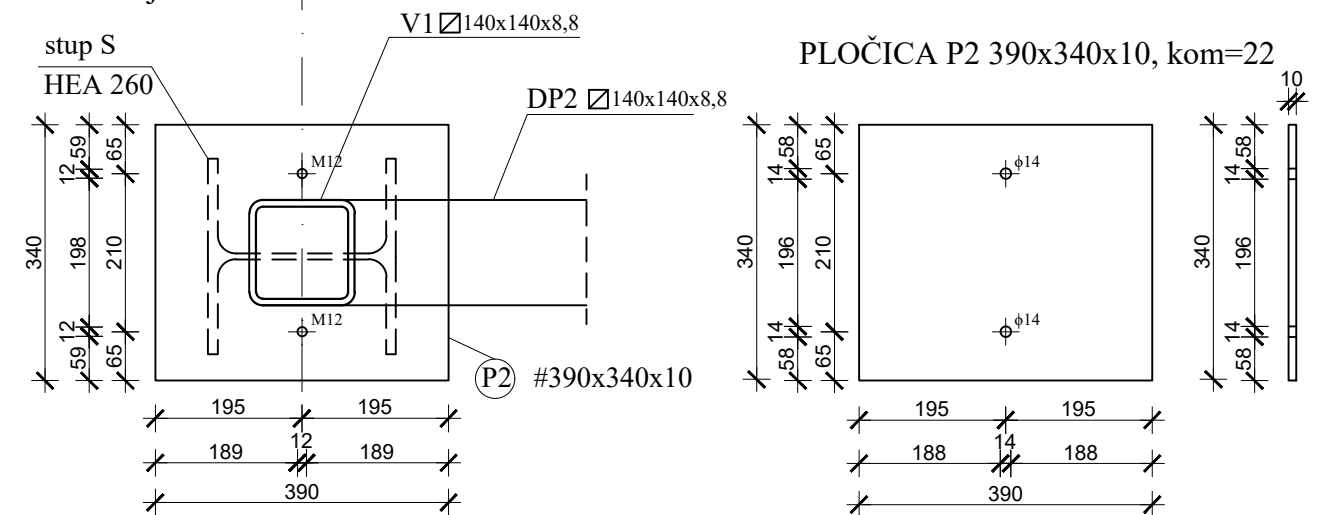
Presjek 2-2
