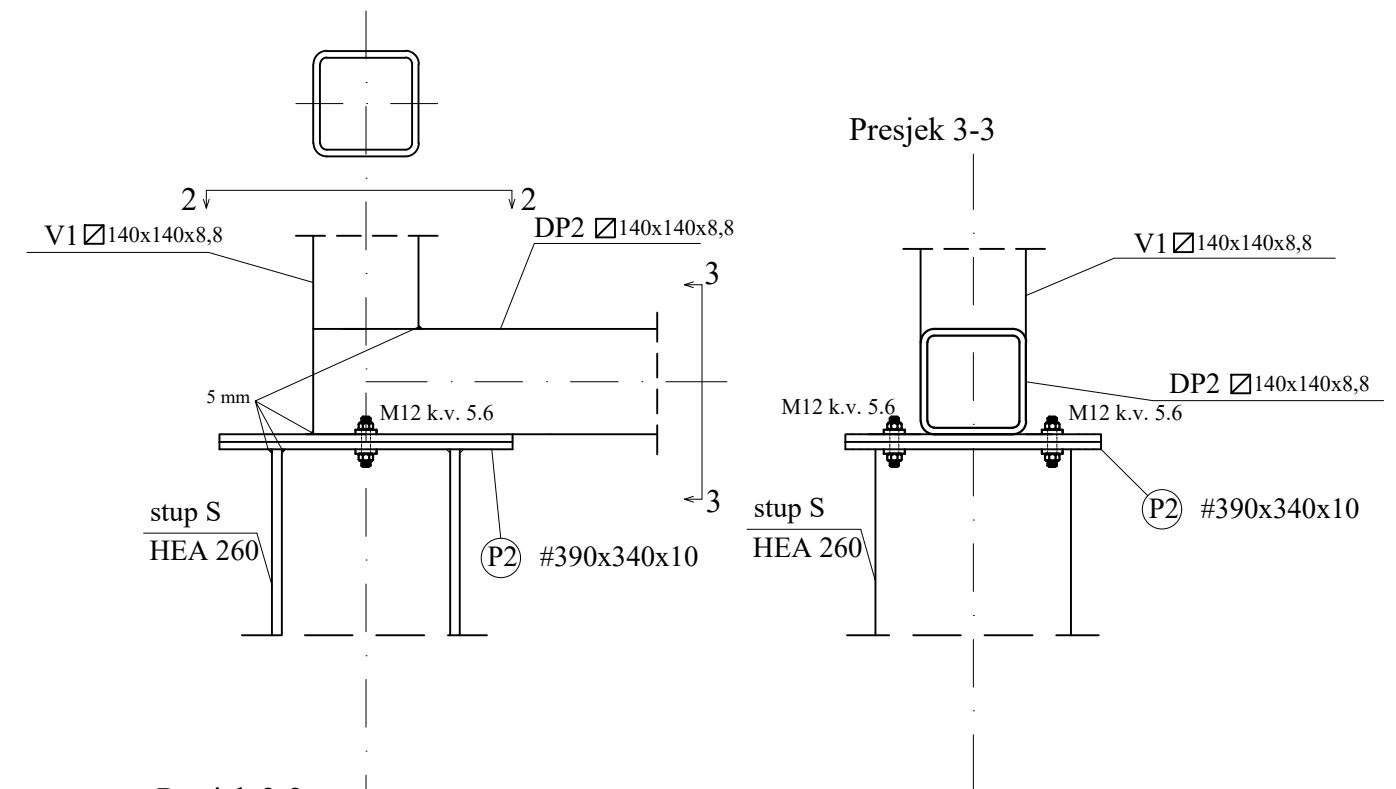
Presjek 2-2
