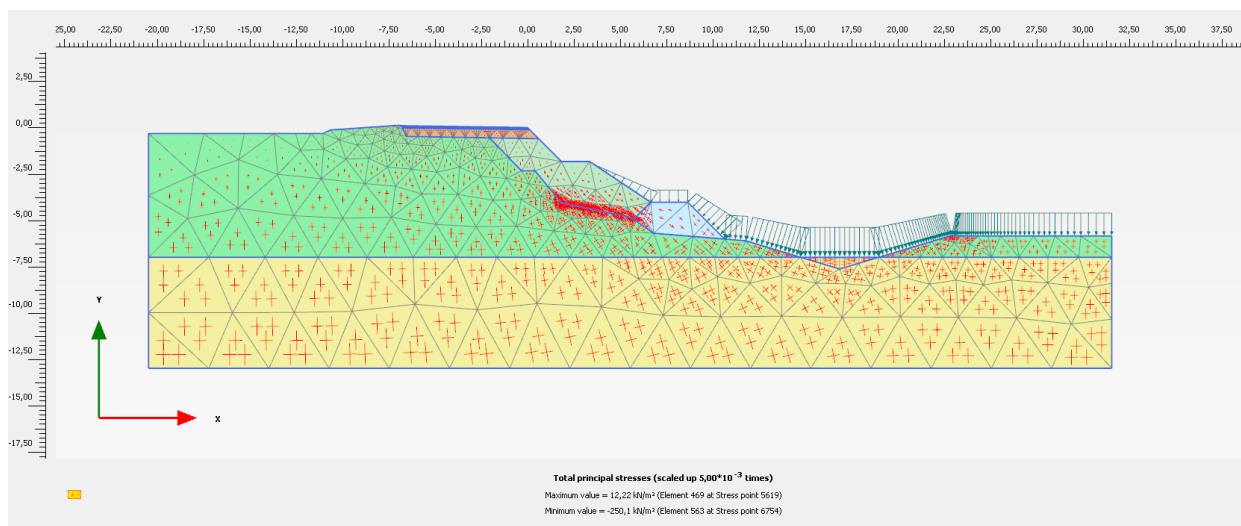
Slika 9. Prikaz djelovanja glavnih naprezanja
