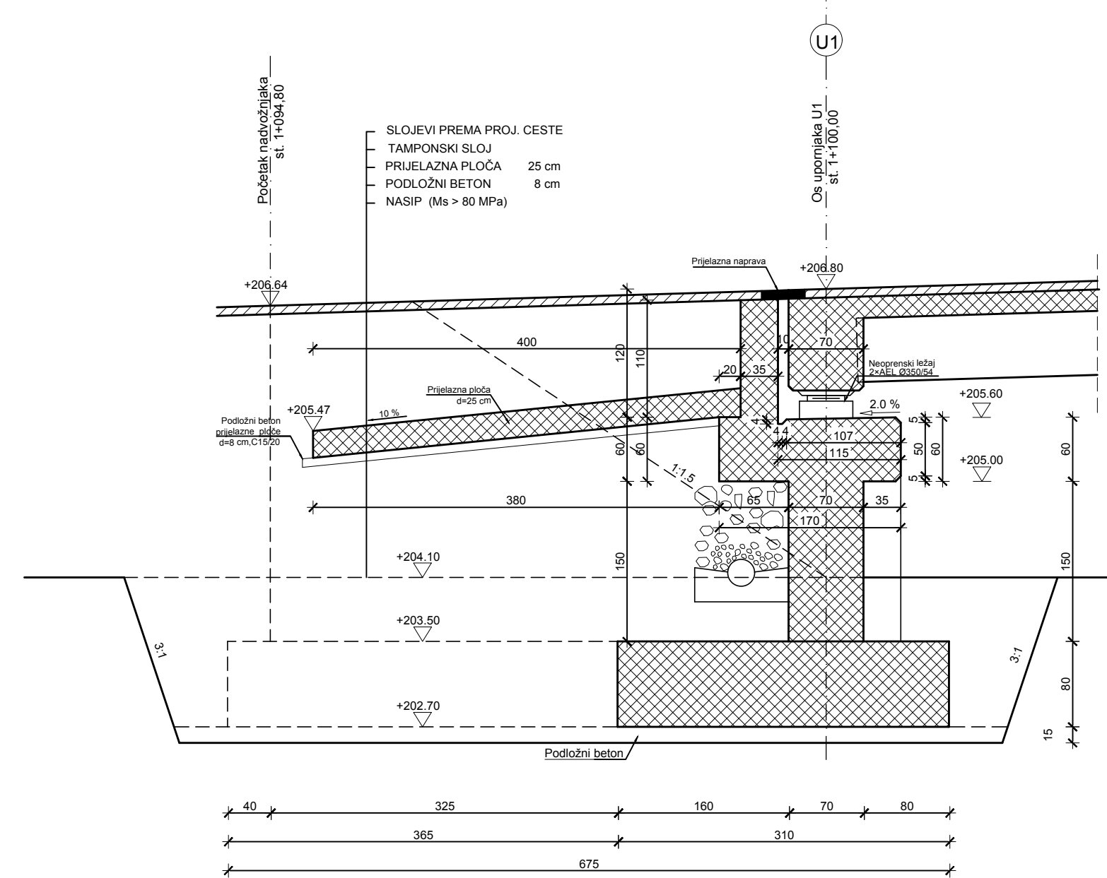
Presjek 2-2
