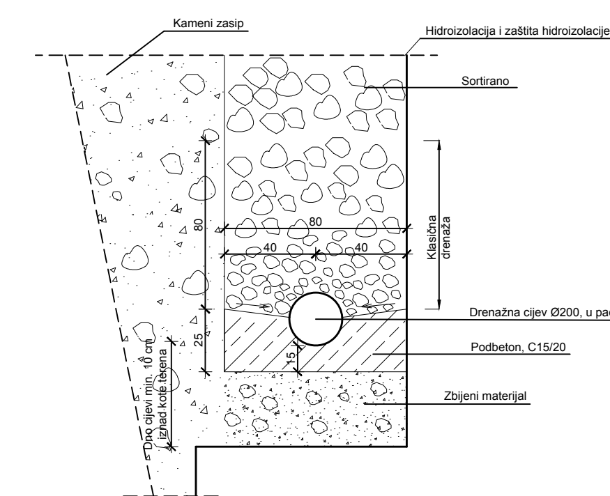
Detalj drenaze
