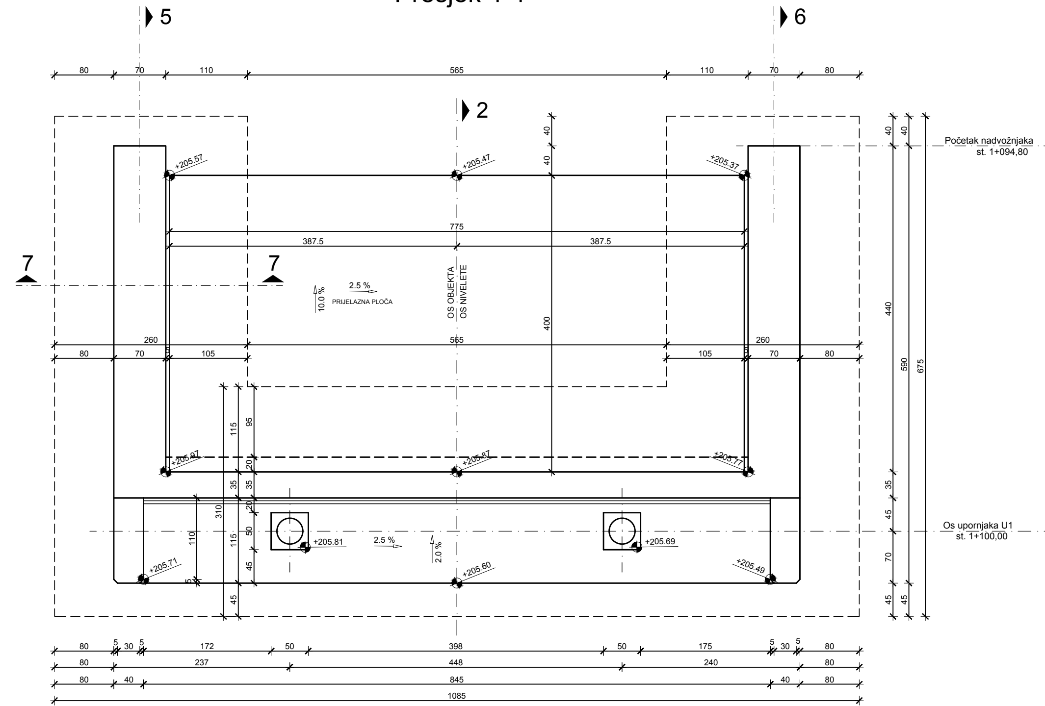
Presjek 4-4
