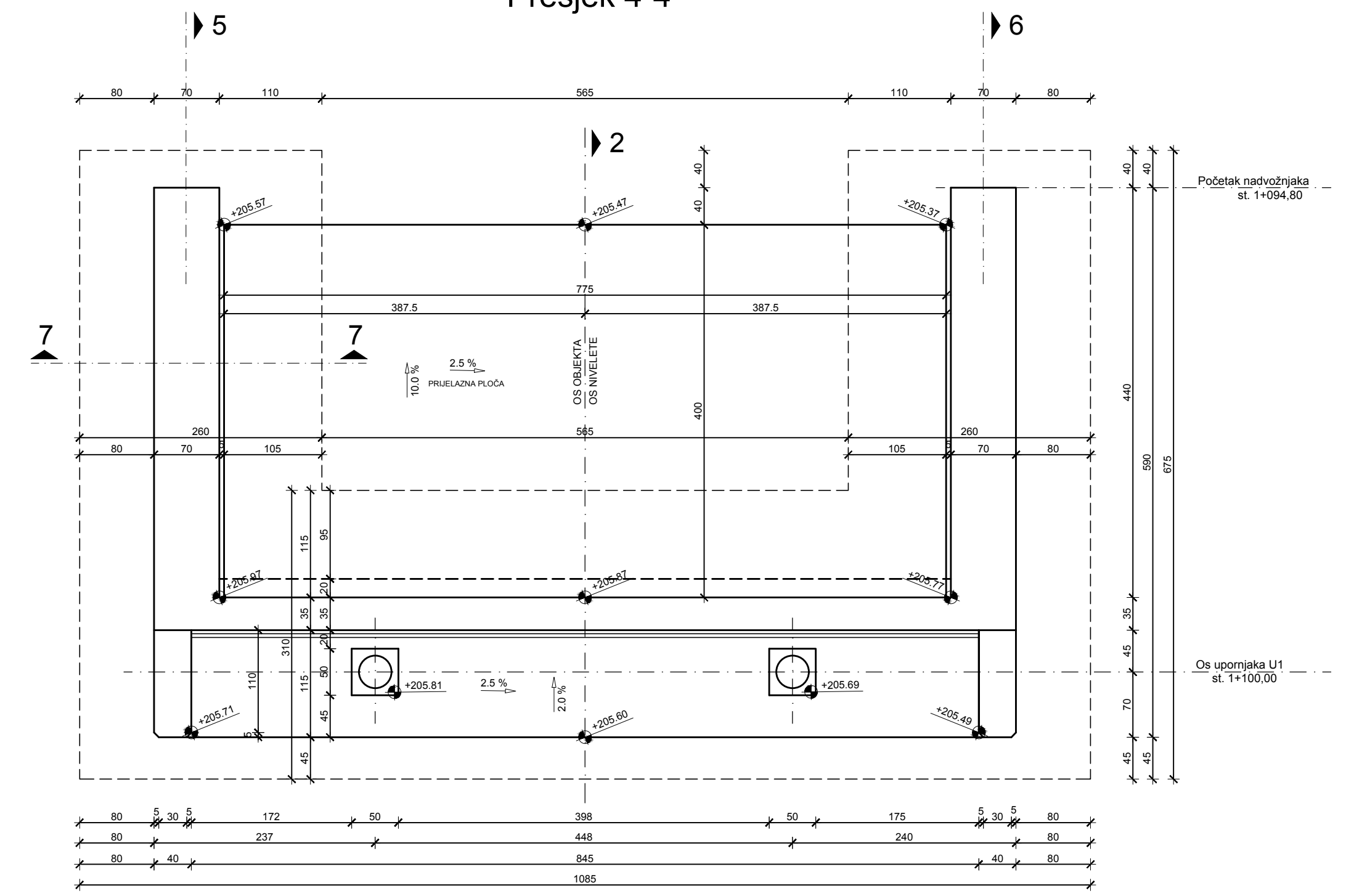
Presjek 4-4
