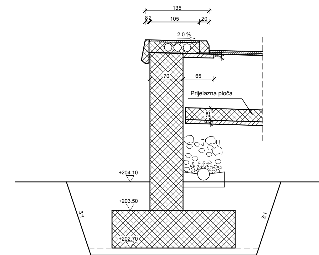
Presjek 7-7
