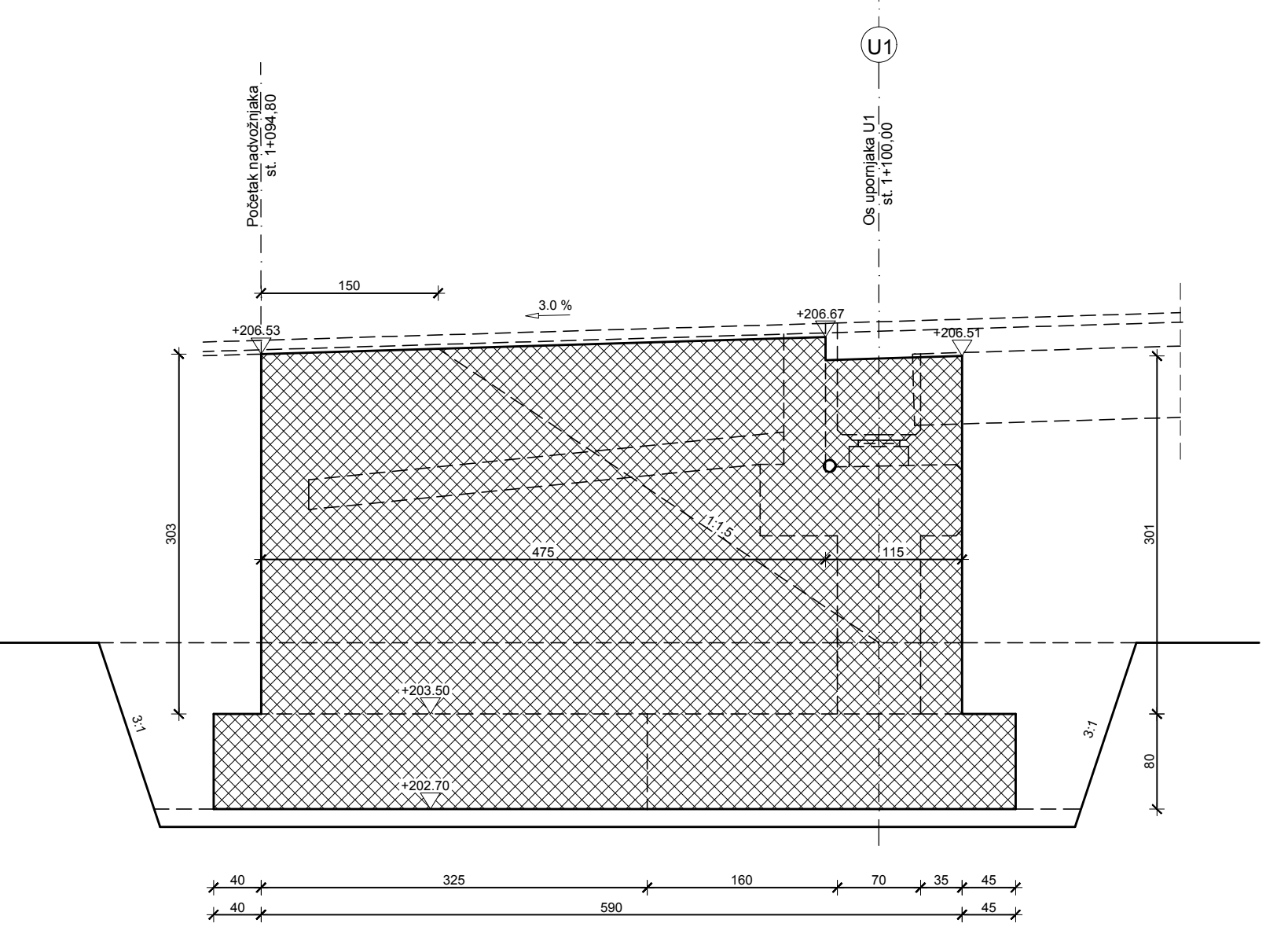
Presjek 6-6
