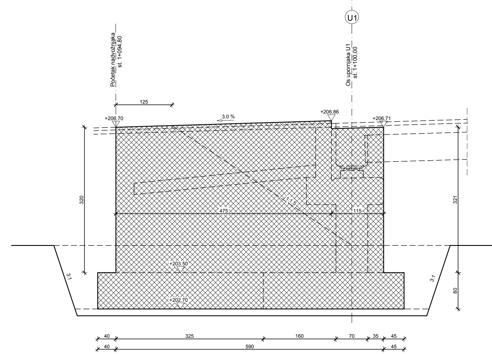
Presjek 5-5
