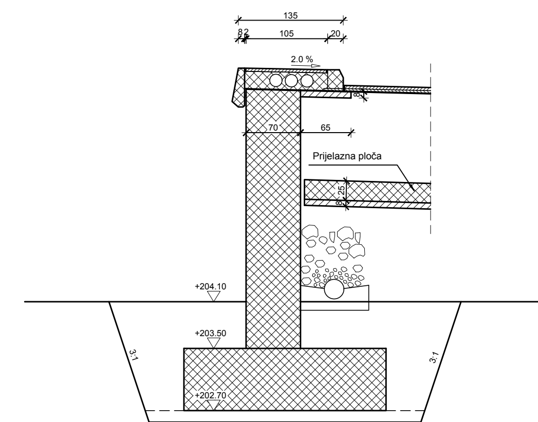
Presjek 7-7
