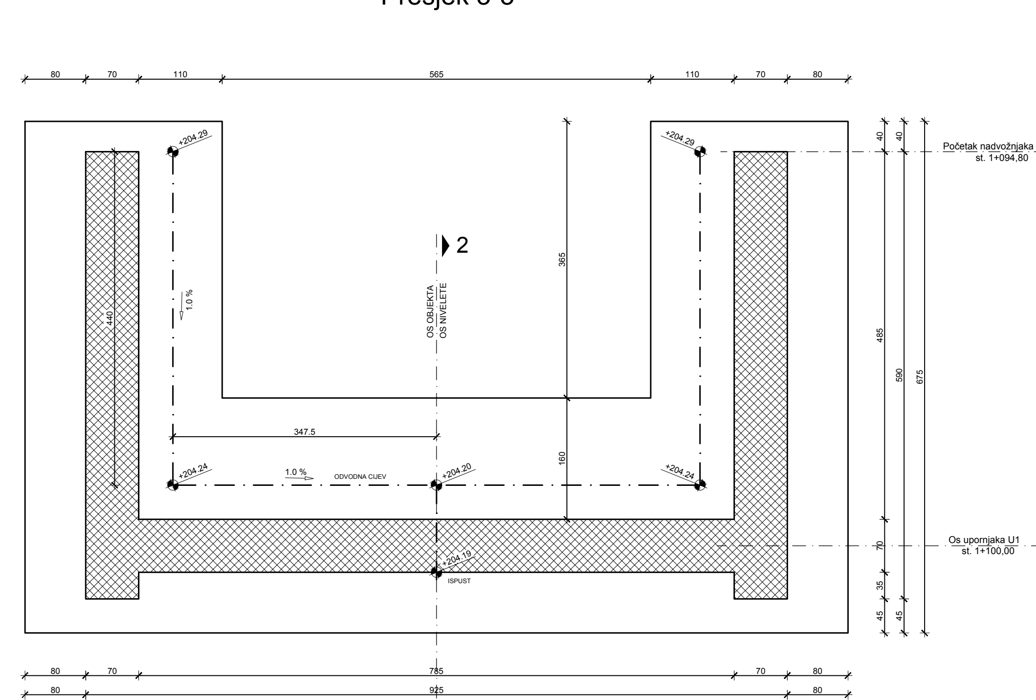
Presjek 3-3
