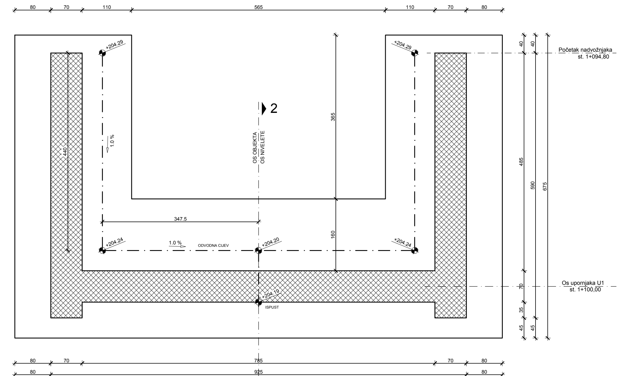
Presjek 3-3
