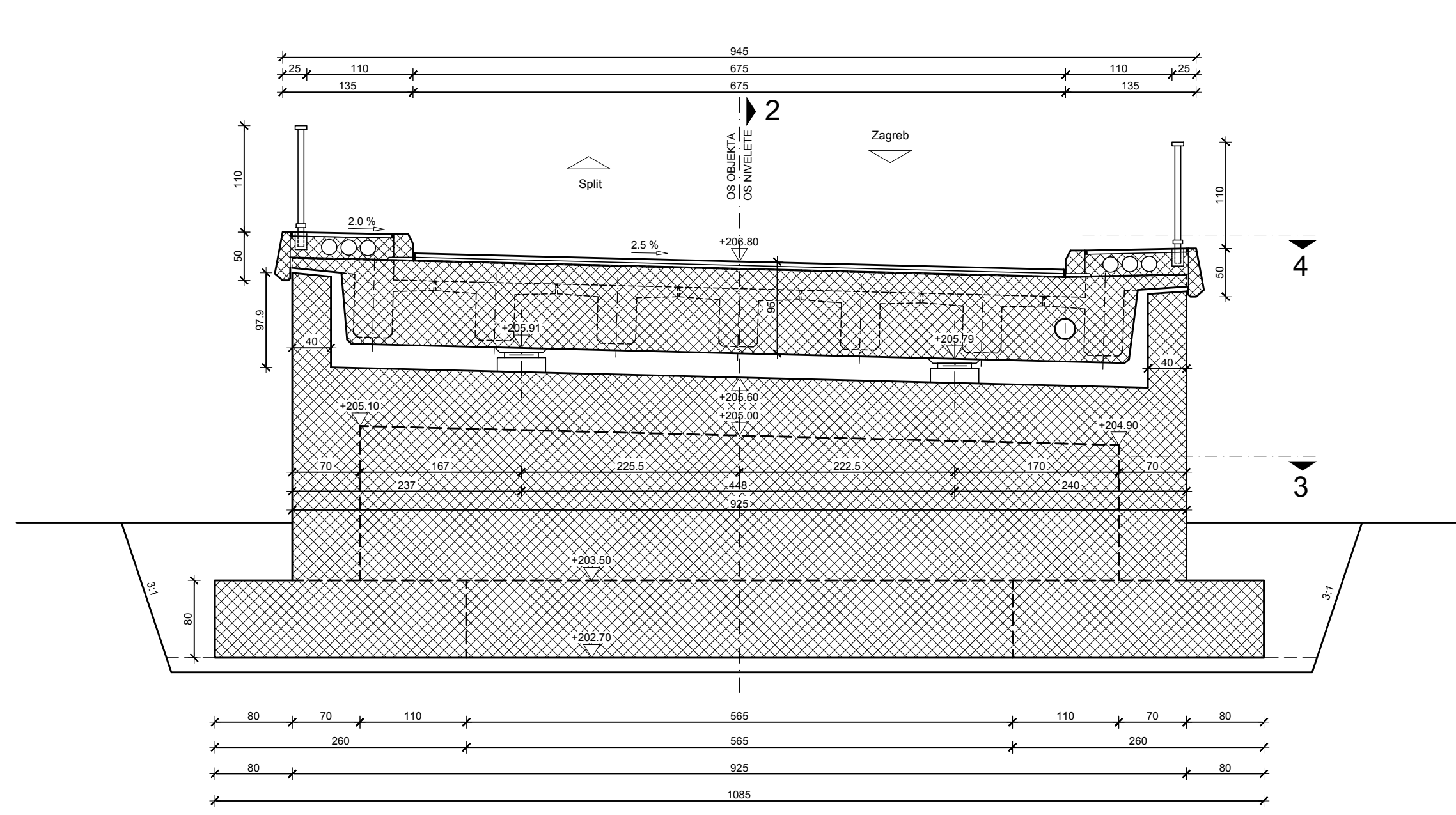
Presjek 1-1
