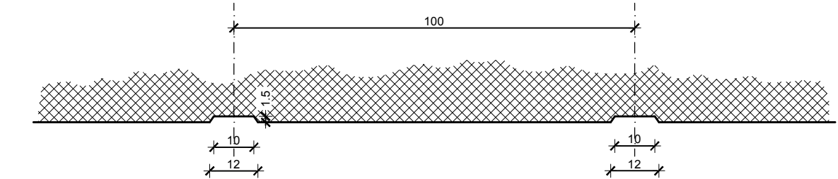
Detalj drenaze
