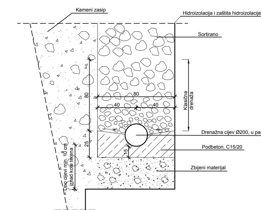
Detalj drenaze
