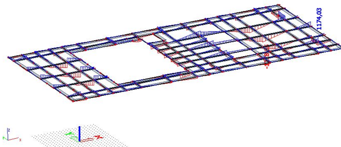
Slika 5.3. Rezne sile-Vz
