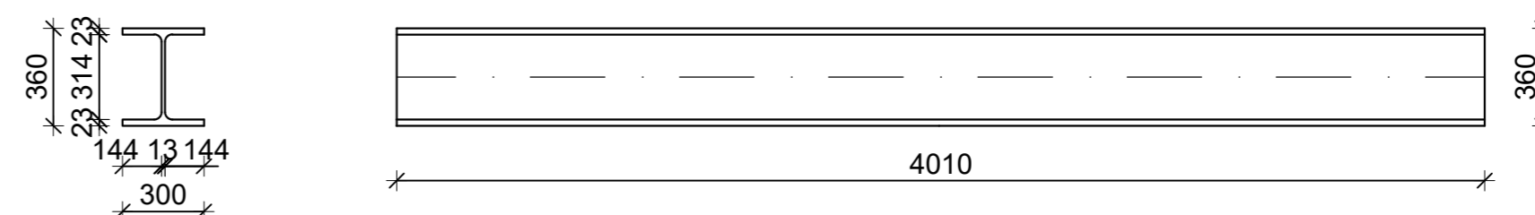
POZ 10 HEB 360
