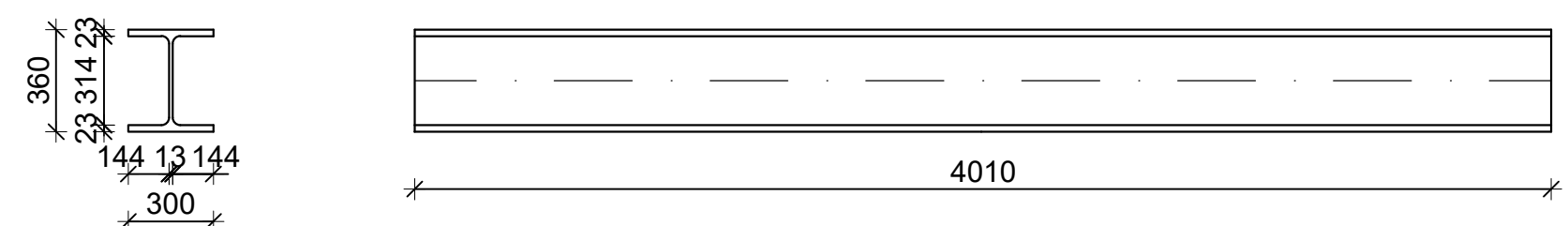
POZ 10 HEB 360
