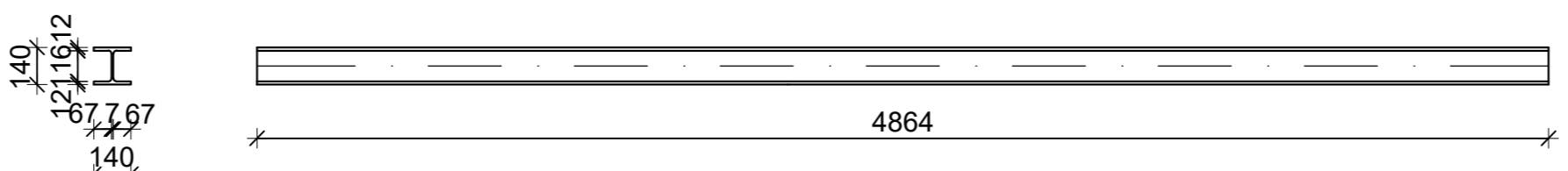
POZ 8 HEB 140
