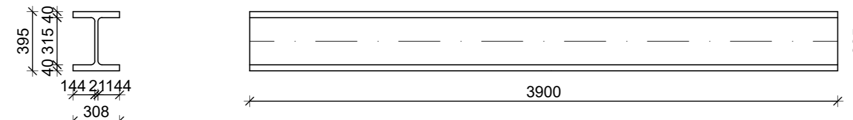
POZ 5 HEM 360
