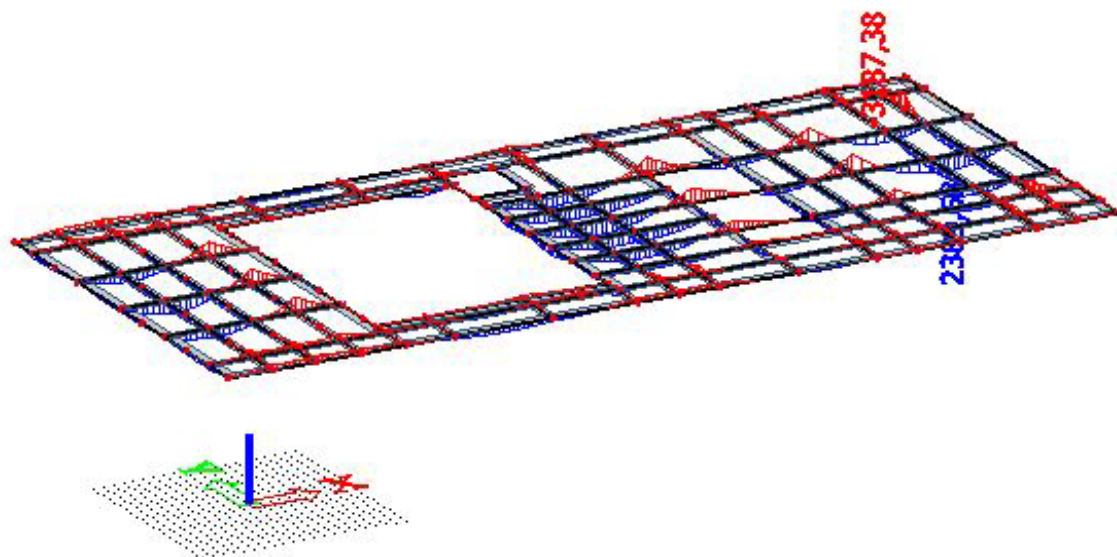
Slika 5.2. Rezne sile-My
