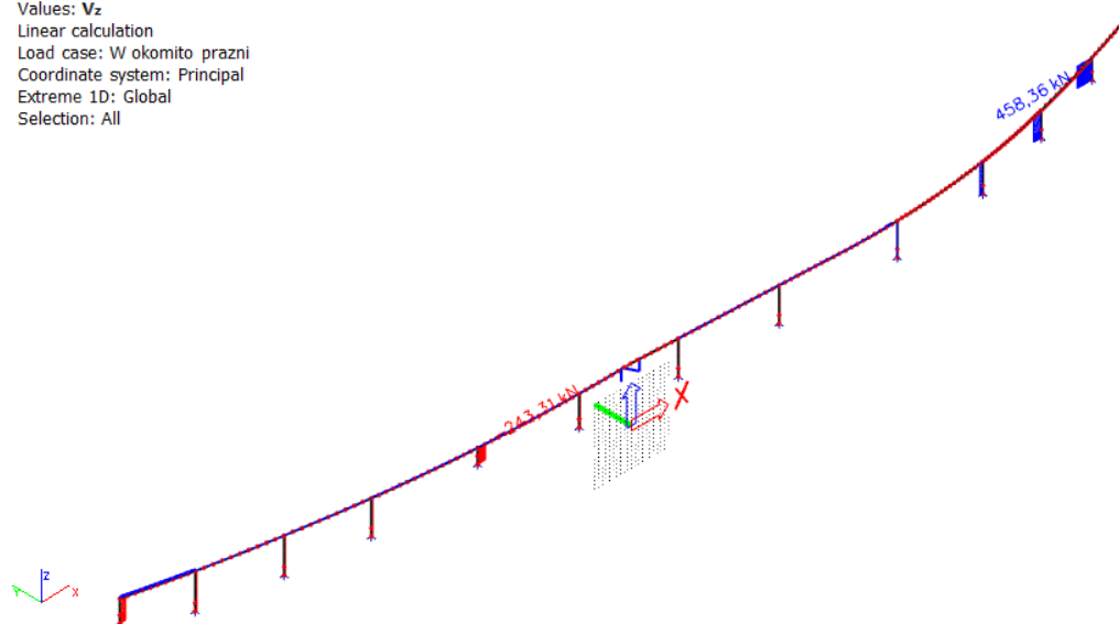
Slika 3.54 Poprečna sila V_z
