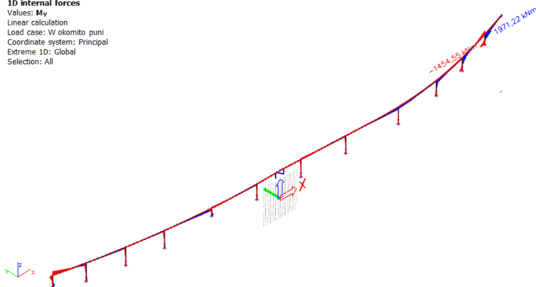
Slika 3.49 Moment savijanja M_y
