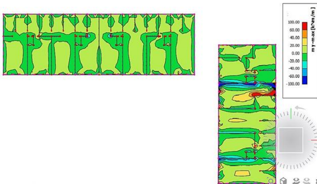
Slika 10.18. Prikaz momenata savijanja – m_y
