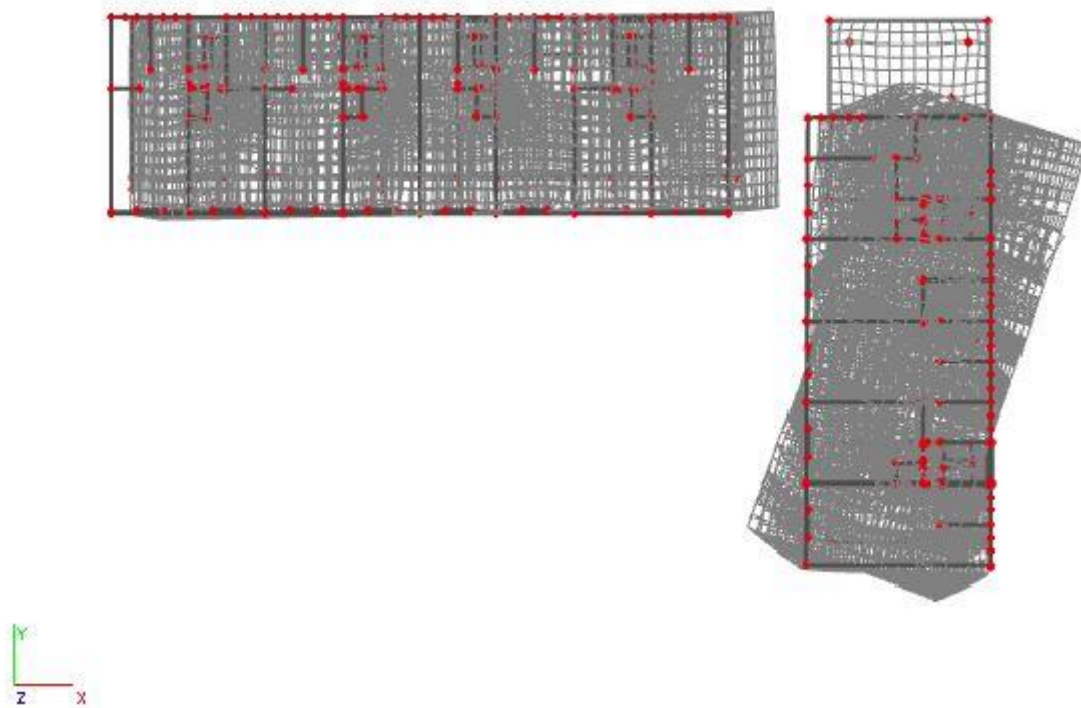
Slika 8.26 Torzija oko globalne osi z -3.mod(prikaz oko osi Z)
