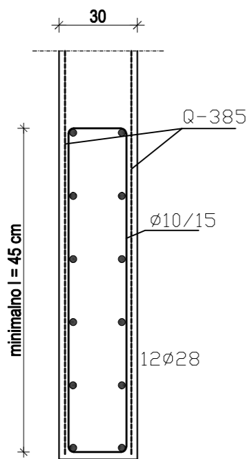
Detalj A
