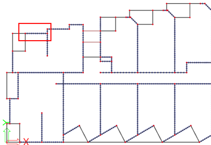
Slika 9.1. Prikaz karakterističnog zida za koji će se vršiti proračun
