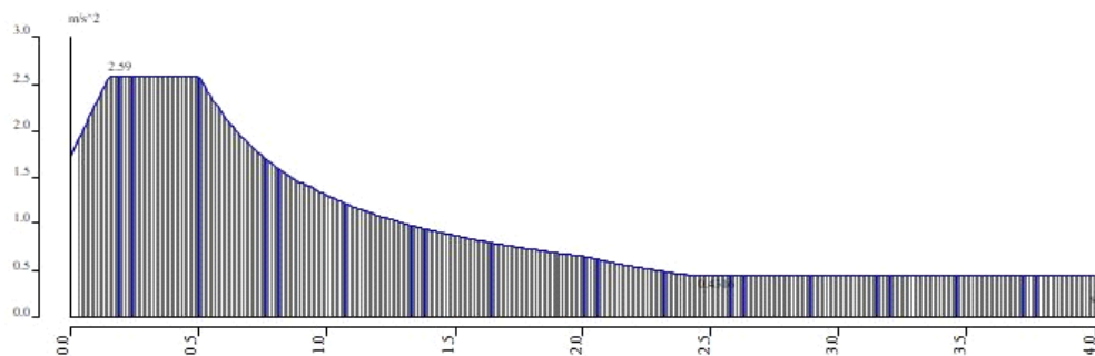
Slika 3.2. Spektar odziva korišten u programu SCIA Engineer 18.1
