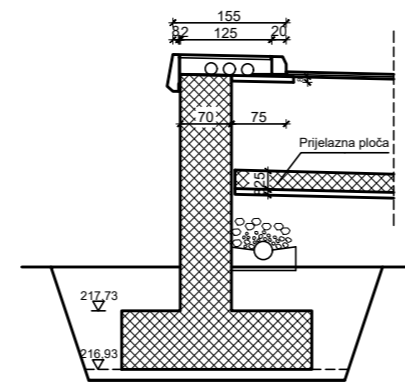
PRESJEK 7-7
