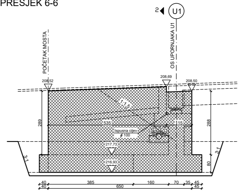
PRESJEK 6-6
