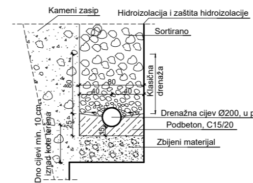
DETALJ DRENAŽE
