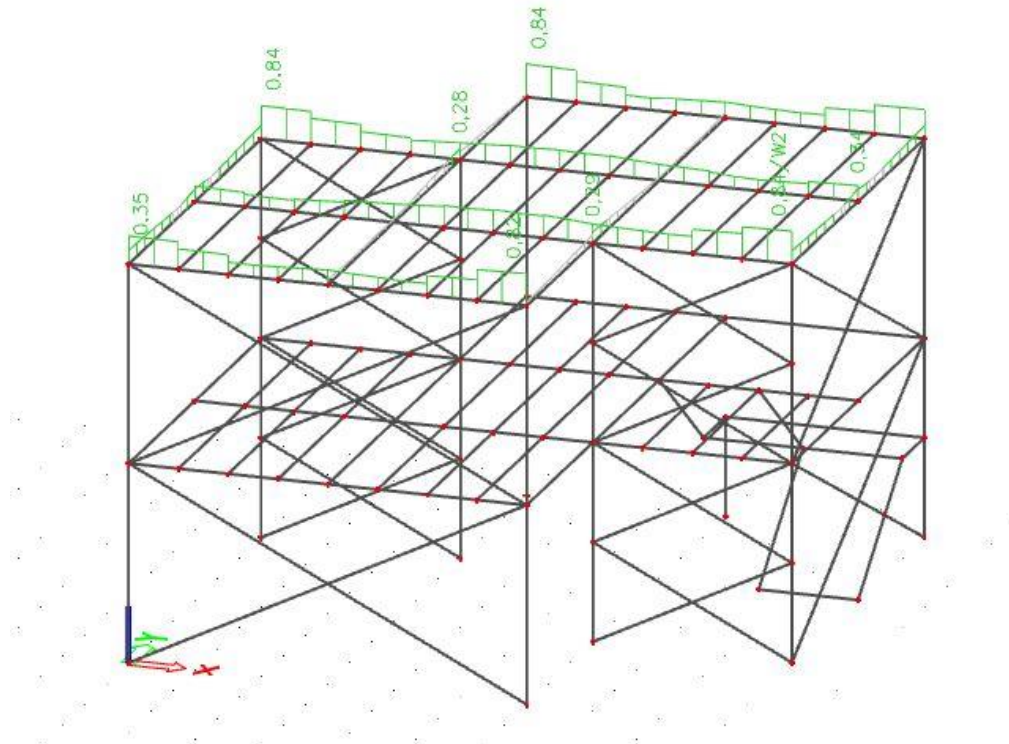
Prikaz iskoristivosti glavnih krovnih greda
