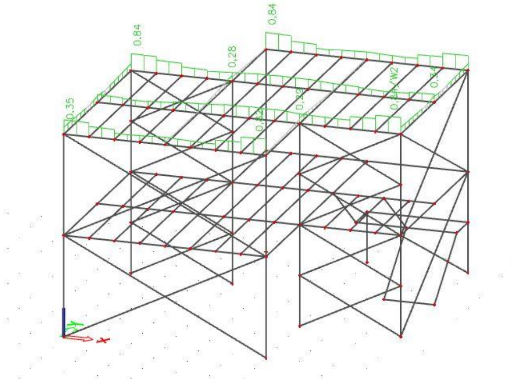
Prikaz iskoristivosti glavnih krovnih greda
