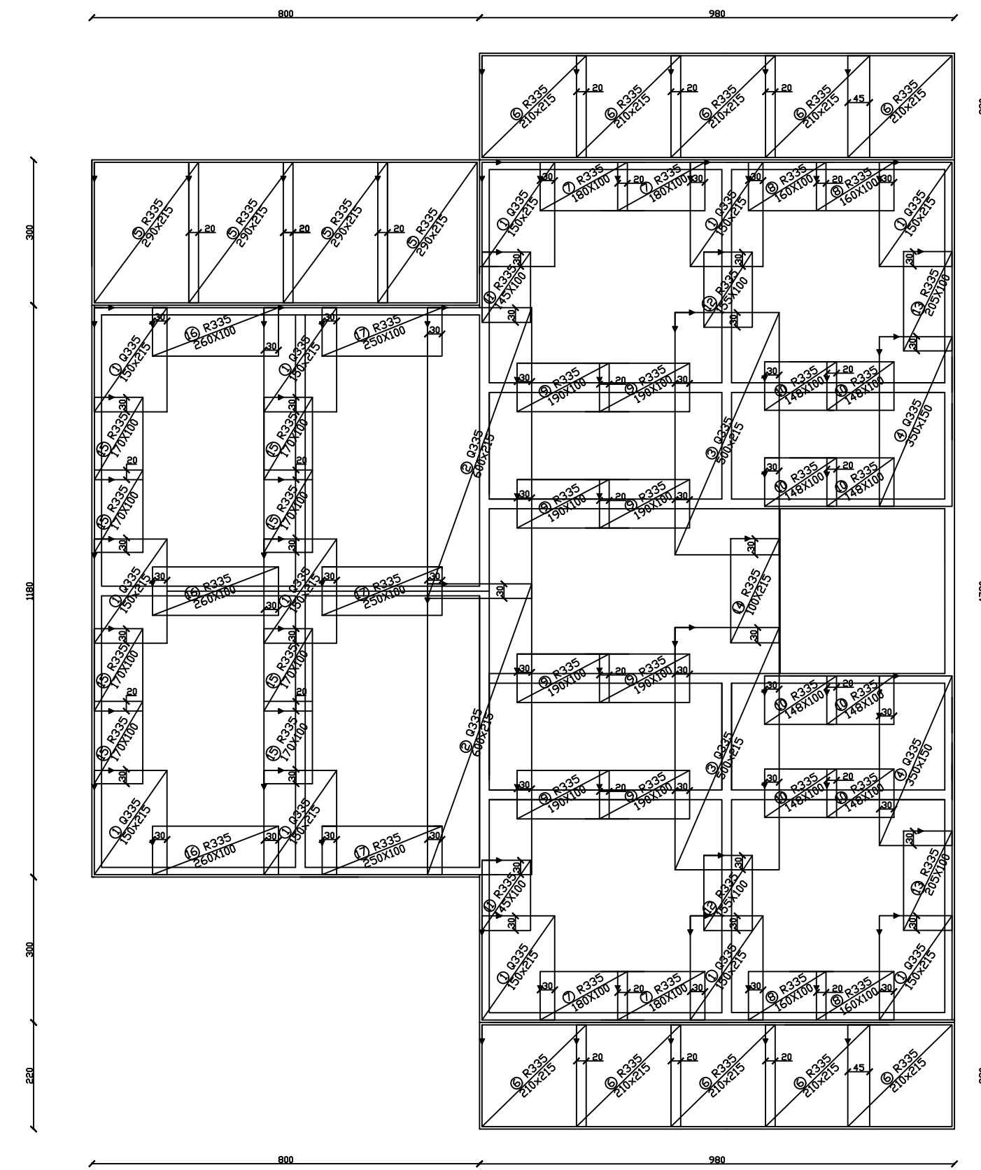
PLAN ARMATURE POZICIJE 200 - GORNJA ZONA
