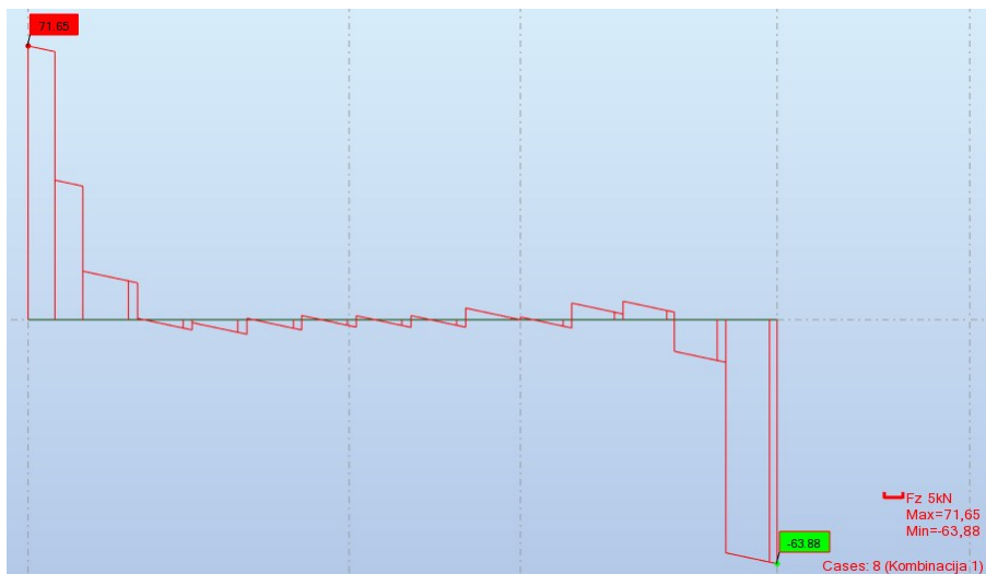
Slika 4.2. Poprečna sila grede POZ 101
