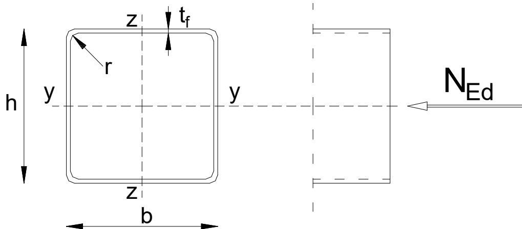
Slika 47 Poprečni presjek gornjeg pojasa
