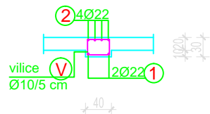
PRESJEK 1-1
