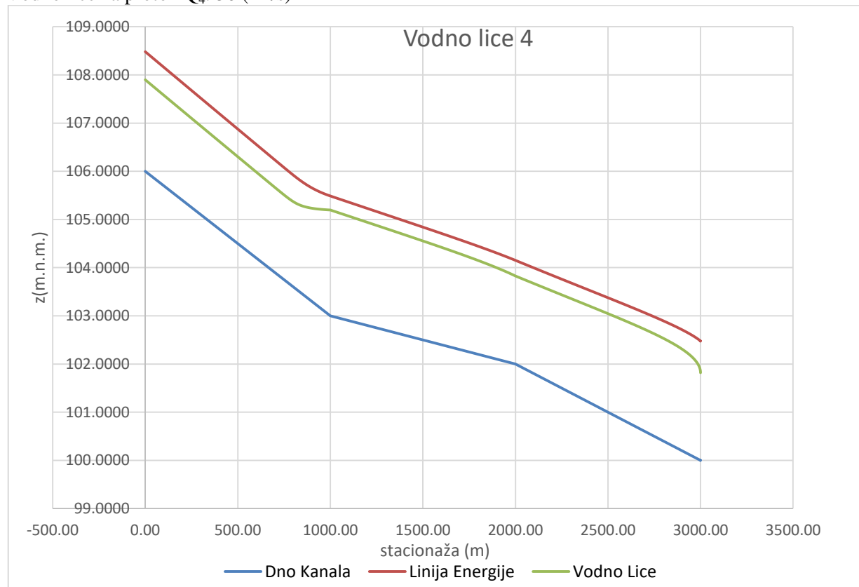
Dijagram 4. Vodno lice za protok Q_4
