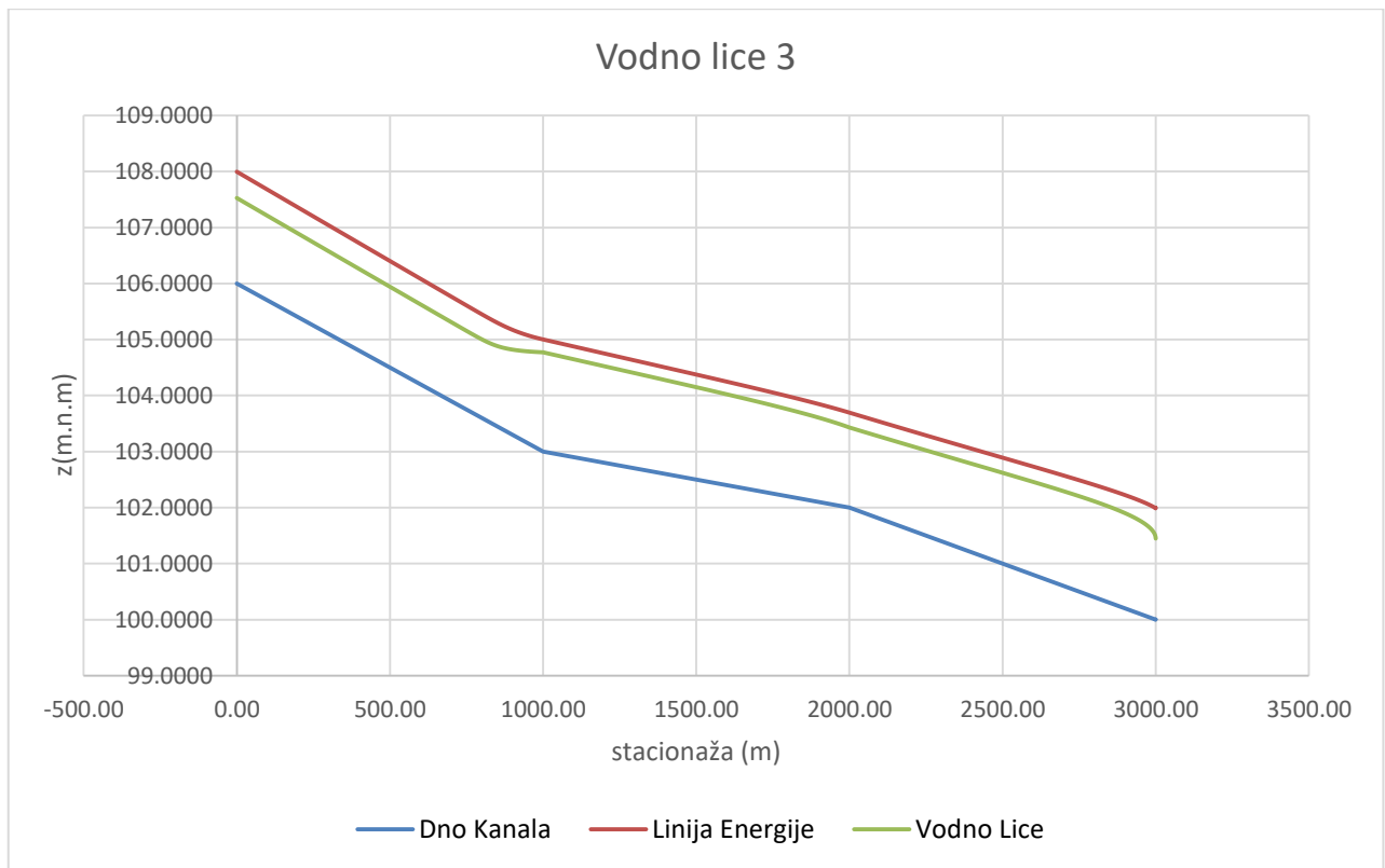
Dijagram 3. Vodno lice za protok Q_3
