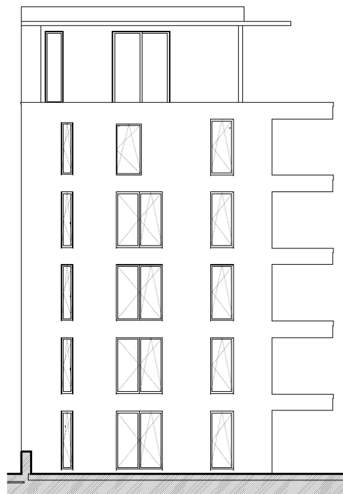
Slika 1.5 Zapadno pročelje
