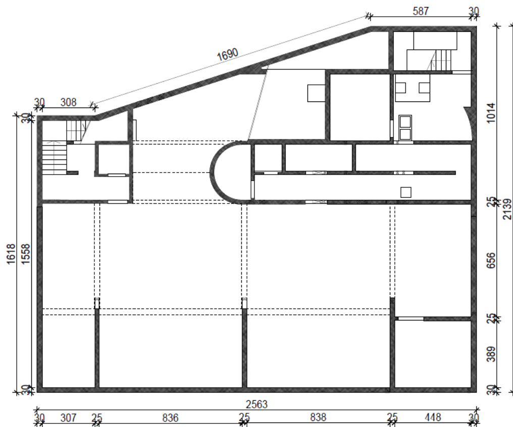
Slika 1.6 Tlocrt razine -2
