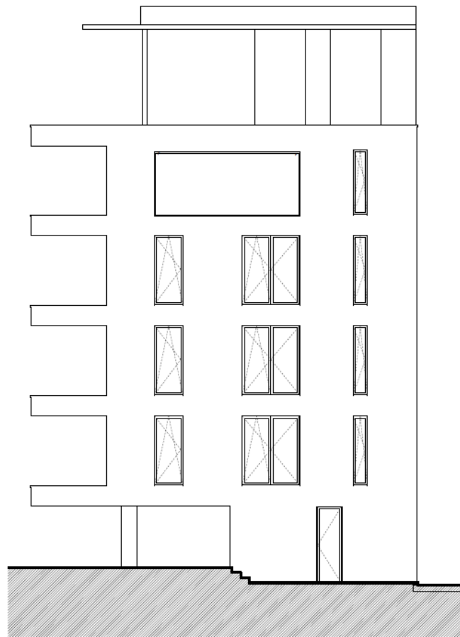
Slika 1.4 Istočno pročelje
