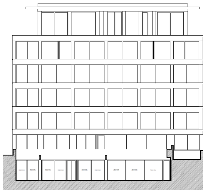
Slika 1.3 Južno pročelje
