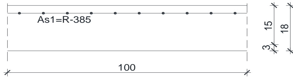
Slika 10.30 Skica armature ploče na ležaju
