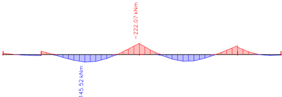
Slika 10.32 Maksimalni momenti savijanja M_y
