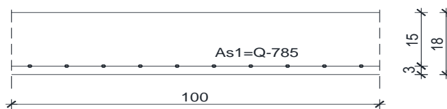
Slika 10.26 Skica armature ploče u polju
