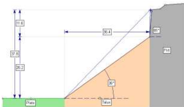
(a) Geometrija zasjeka bez barijere.
