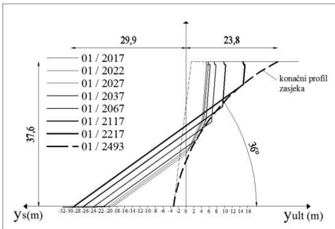
Slika 19. Promjena geometrije lica zasjeka u vremenu
