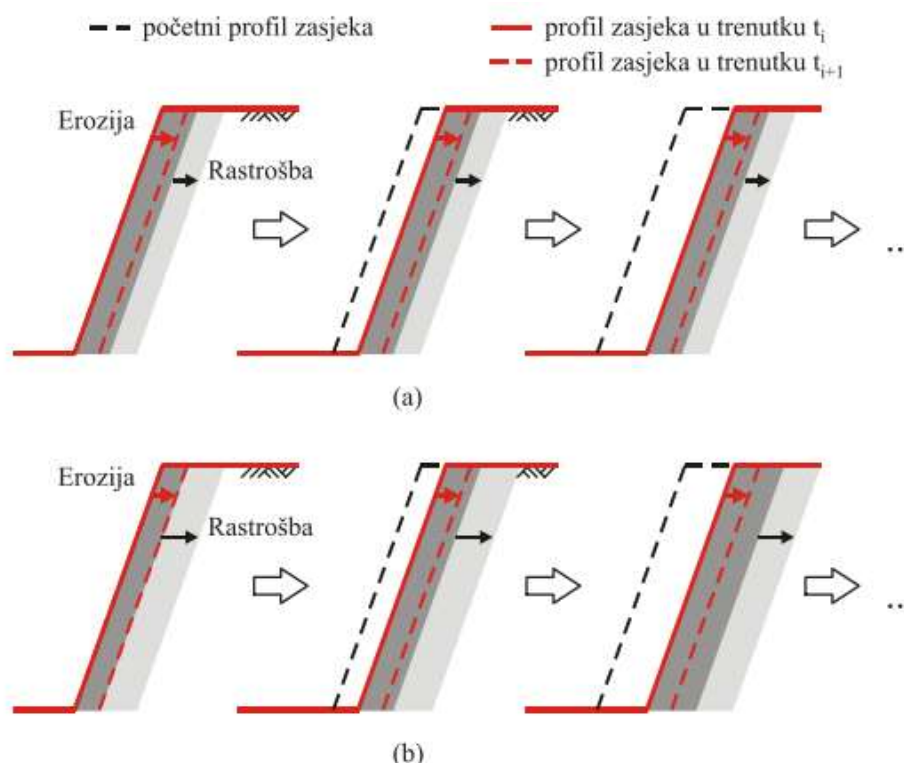
Slika 11. Vremenski tok promjene profila zasjeka za slučaj: a) ravnoteža erozije i rastrošbe; b) neravnoteže u korist rastrošbe (svijetlo sivo-rastrošeni materijal, tamno sivo-ostatak iz prethodnog intervala) [18]
