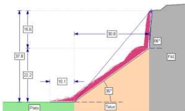
(c) Trajektorije blokova bez barijere.
