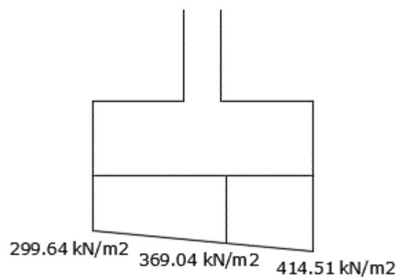
Slika 14.5 Prikaz naprezanja
