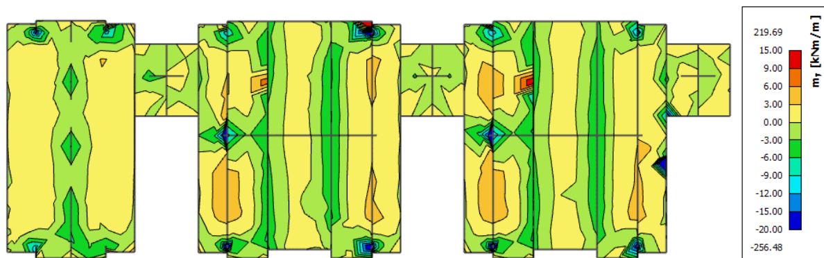
Slika 11.61 Prikaz momenata savijanja – m_y
