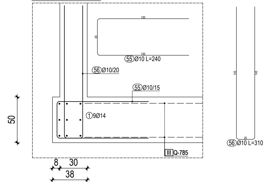
DETALJ 2-2 M 1:25
