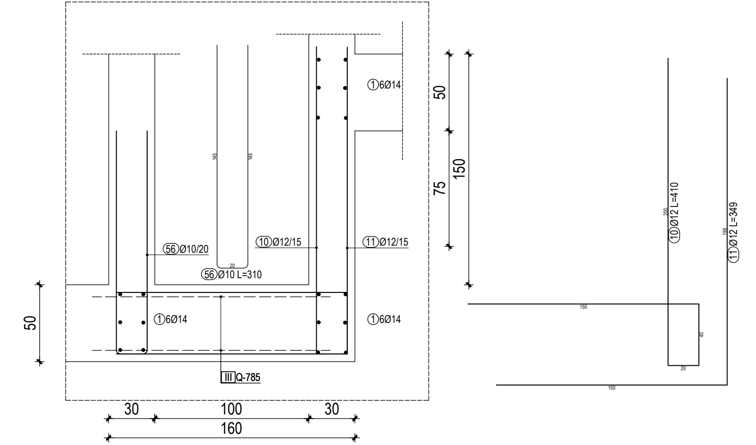
DETALJ 2-2 M 1:25
