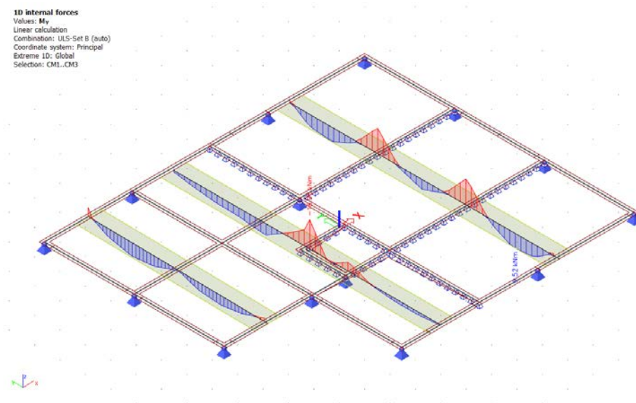
Slika 47 1D dijagram momenata savijanja M_y (kraci smjer)
