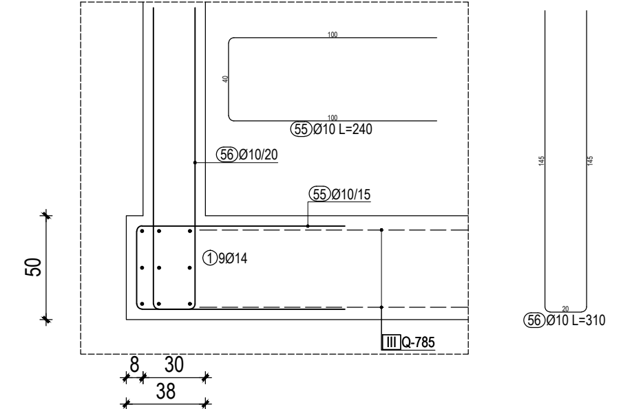
DETALJ 2-2 M 1:25
