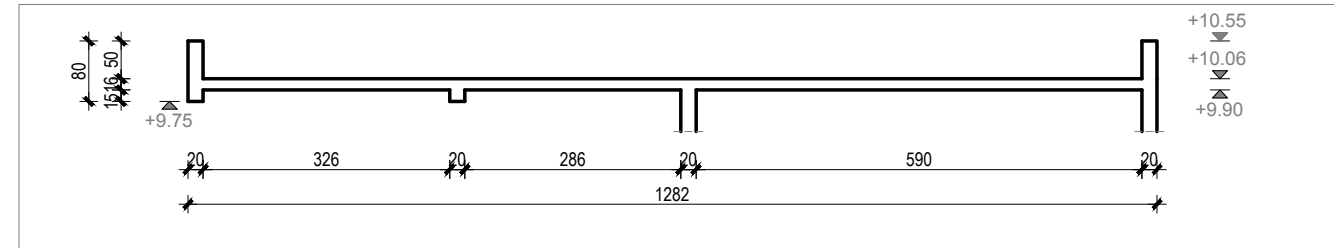
PRESJEK 1-1
