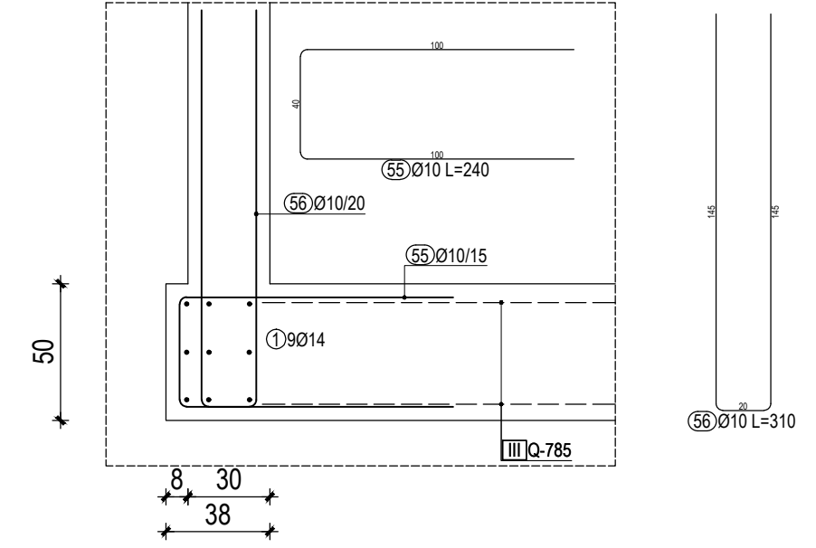
DETALJ 2-2 M 1:25
