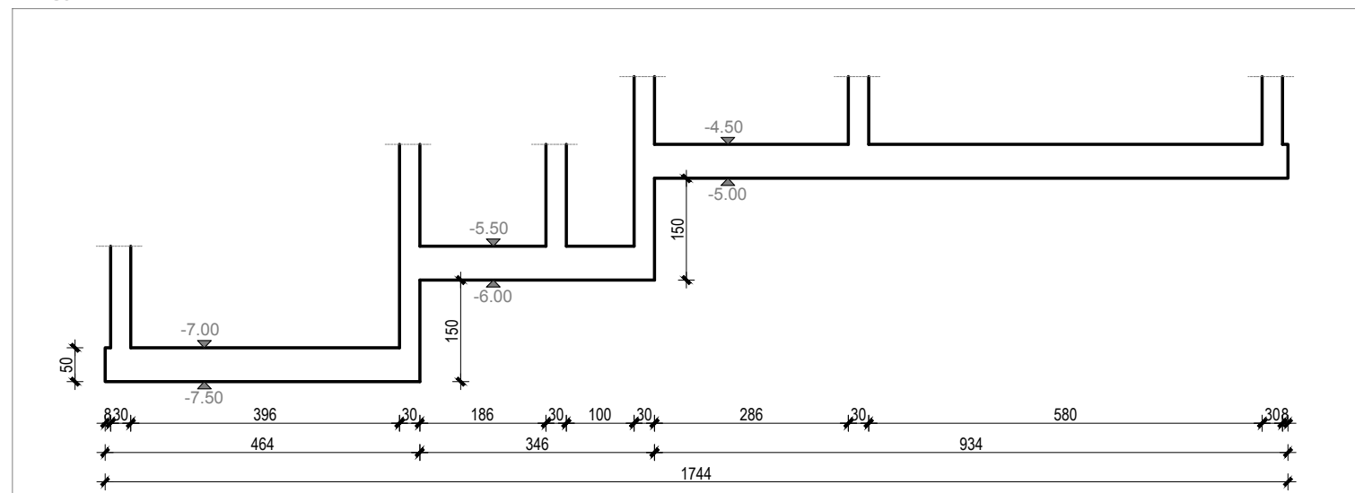
PRESJEK 1-1
