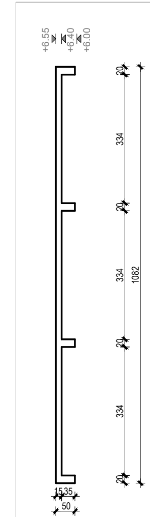
PRESJEK 2-2
