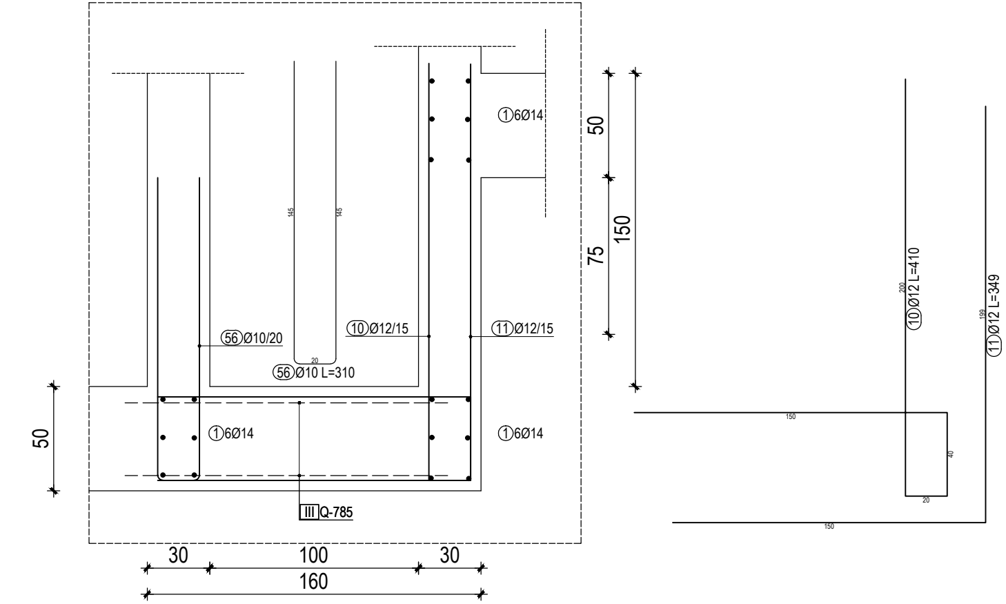
DETALJ 2-2 M 1:25
