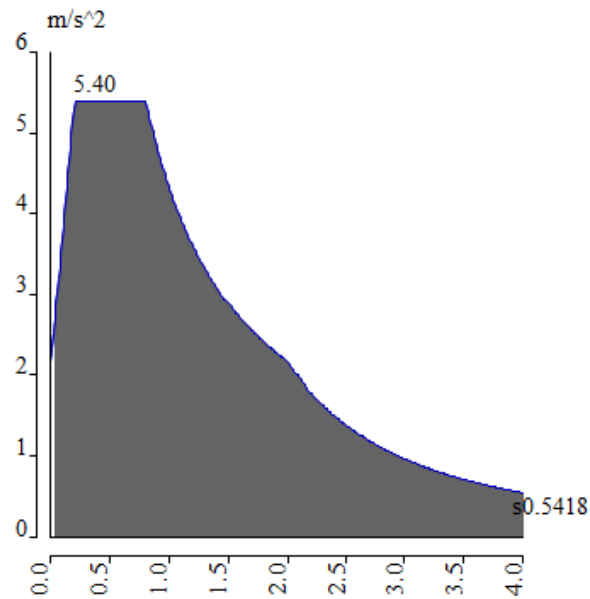
Slika 30 Proračunski spektralni ubrzanja za unesene podatke
