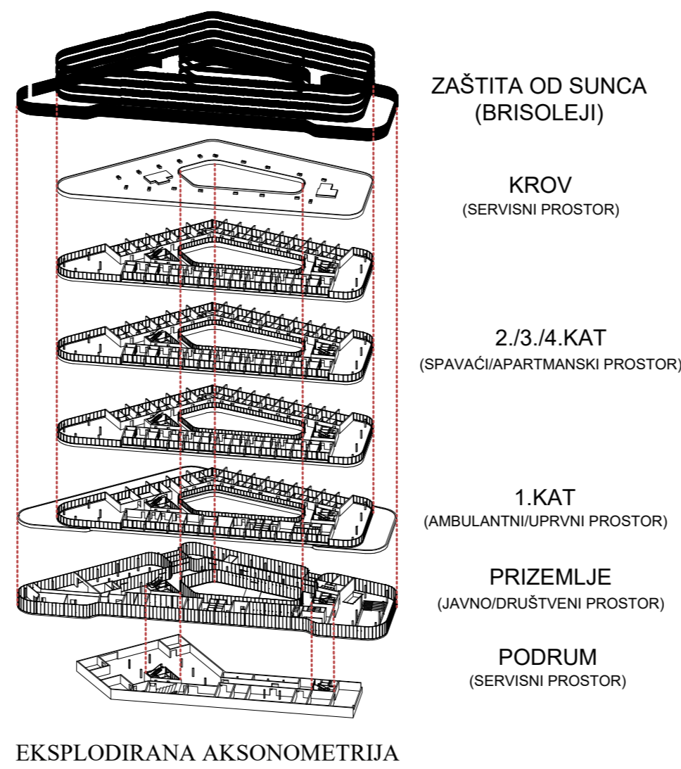
EKSPLODIRANA AKSONOMETRIJA
