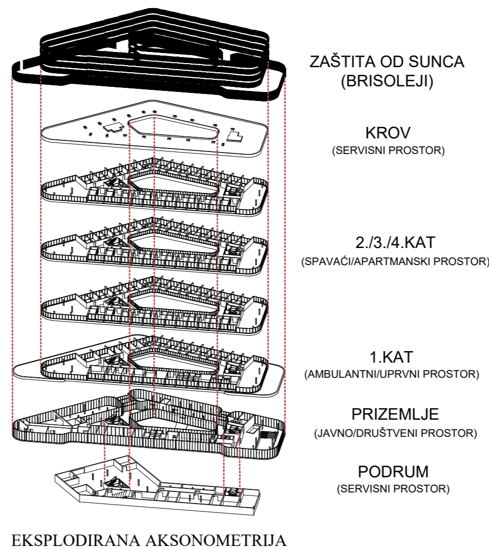
EKSPLODIRANA AKSONOMETRIJA
