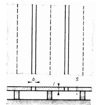
Konstrukcija rezonatora s rasporom
