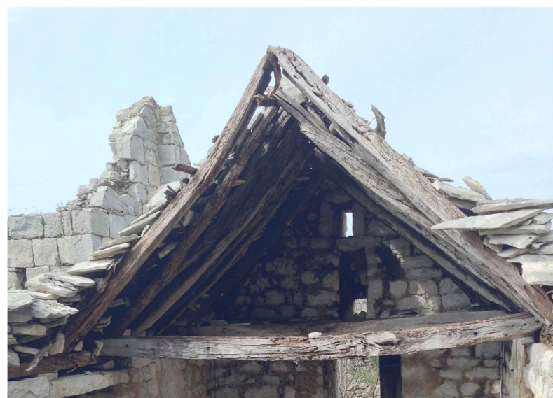
Grafički prilog 52. Propalo krovište uslijed opterećenja kamenom, Gata
