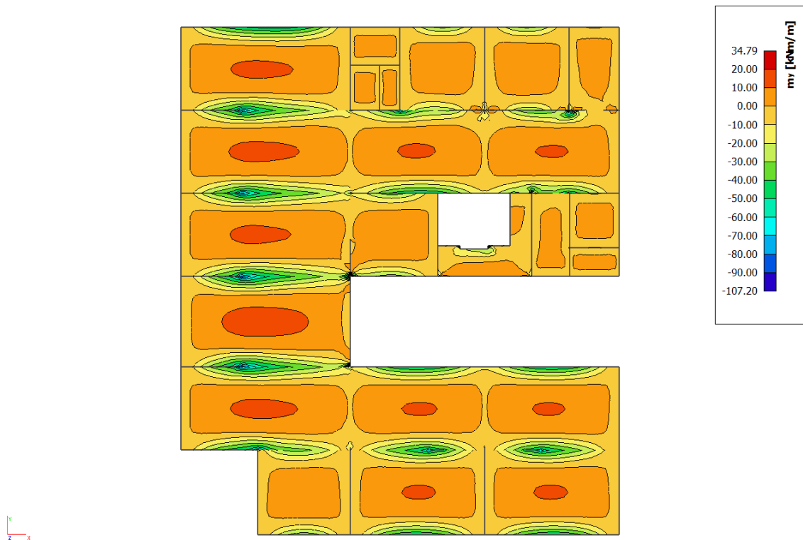
Slika 6.55. Dijagram momenata savijanja M_y [ \text{kNm/m} ']
