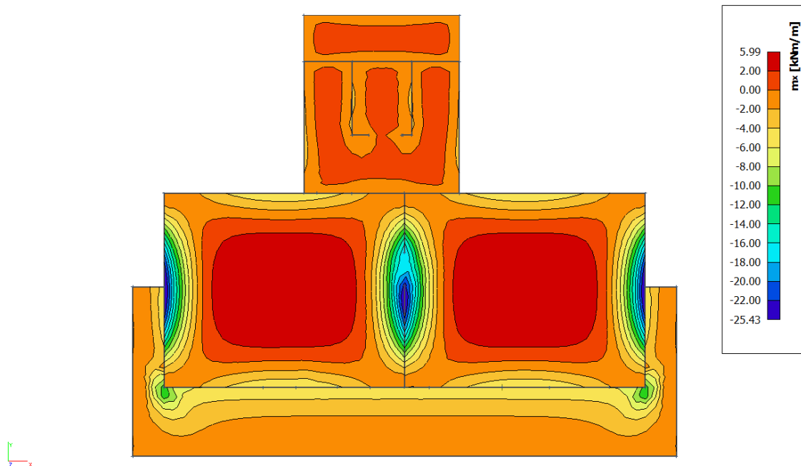
Slika 6.4. Dijagram momenata savijanja M_x [ \text{kNm/m}' ]
