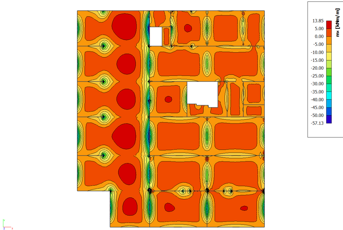
Slika 6.47. Dijagram momenata savijanja M_x [ \text{kNm/m} ']
