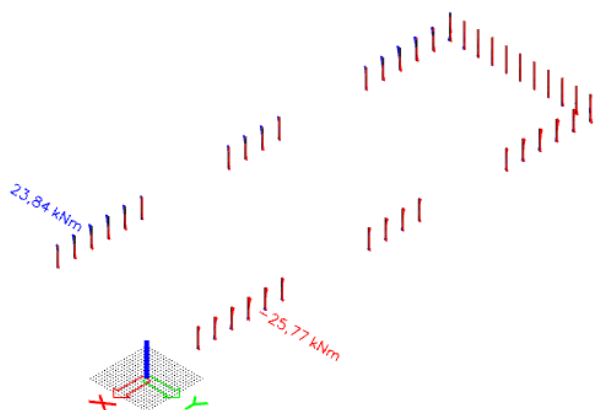
Slika 7.5.5.Moment M_z
