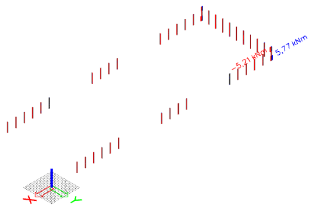
Slika 7.5.3.Moment M_x
