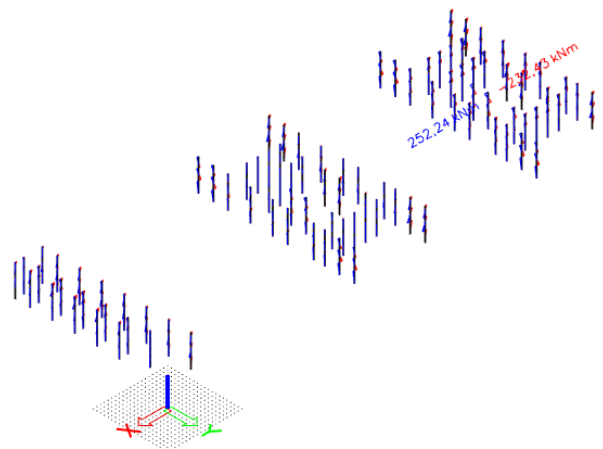
Slika 7.8.5. Moment M_z
