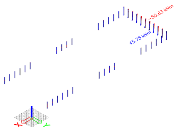
Slika 7.5.3.Moment M_x
