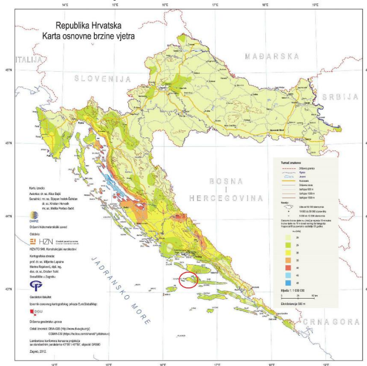
Slika 16 Karta osnovnih brzina vjetra V_{b,0}
