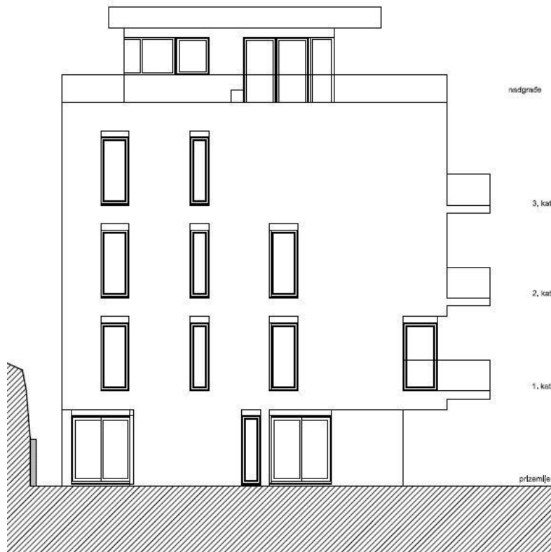
Slika 5 Zapadno pročelje
