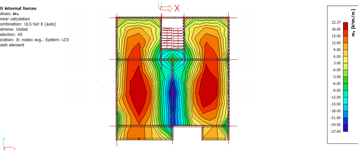
Slika 92 2D dijagram momenata savijanja M_x
