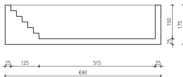
PRESJEK A-A
