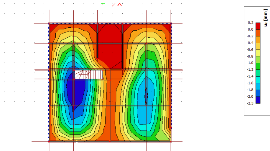
Slika 76 Vrijednost progiba na ploči
