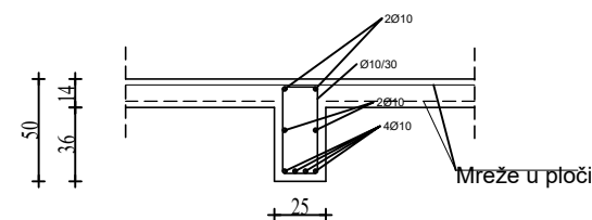
GREDA POZ G704 PRESJEK 5-5 M 1:20
