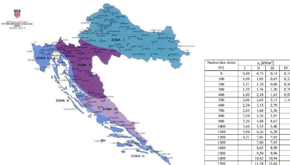
Slika 8.6. Karakteristično opterećenje snijegom s_k (kN/m 2 ) u zonama na različitim nadmorskim visinama
