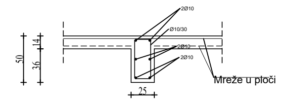
GREDA POZ G704 PRESJEK 6-6 M 1:20
