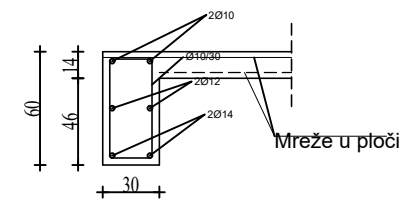
GREDA POZ G703 PRESJEK 4-4 M 1:20
