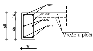
GREDA POZ G702 PRESJEK 0-0 M 1:20
