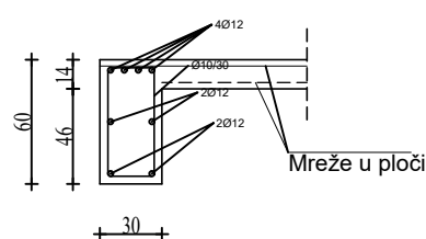
GREDA POZ G702 PRESJEK 2-2 M 1:20
