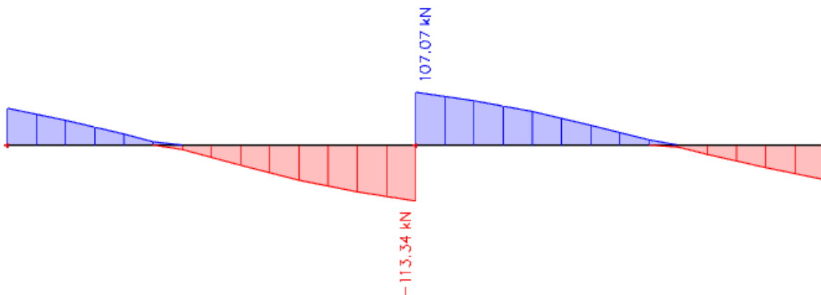
Slika 12.2. Maksimalna poprečna sila V_z
