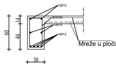
GREDA POZ G702 PRESJEK 1-1 M 1:20
