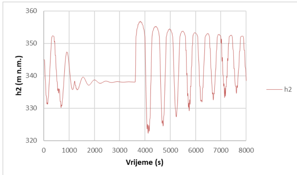
Slika 73 Vodostaj h_2 u ovisnosti o vremenu za Varijantu 3.2
