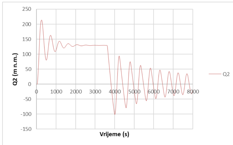
Slika 57 Protok Q2 u ovisnosti o vremenu za Varijantu 2.2
