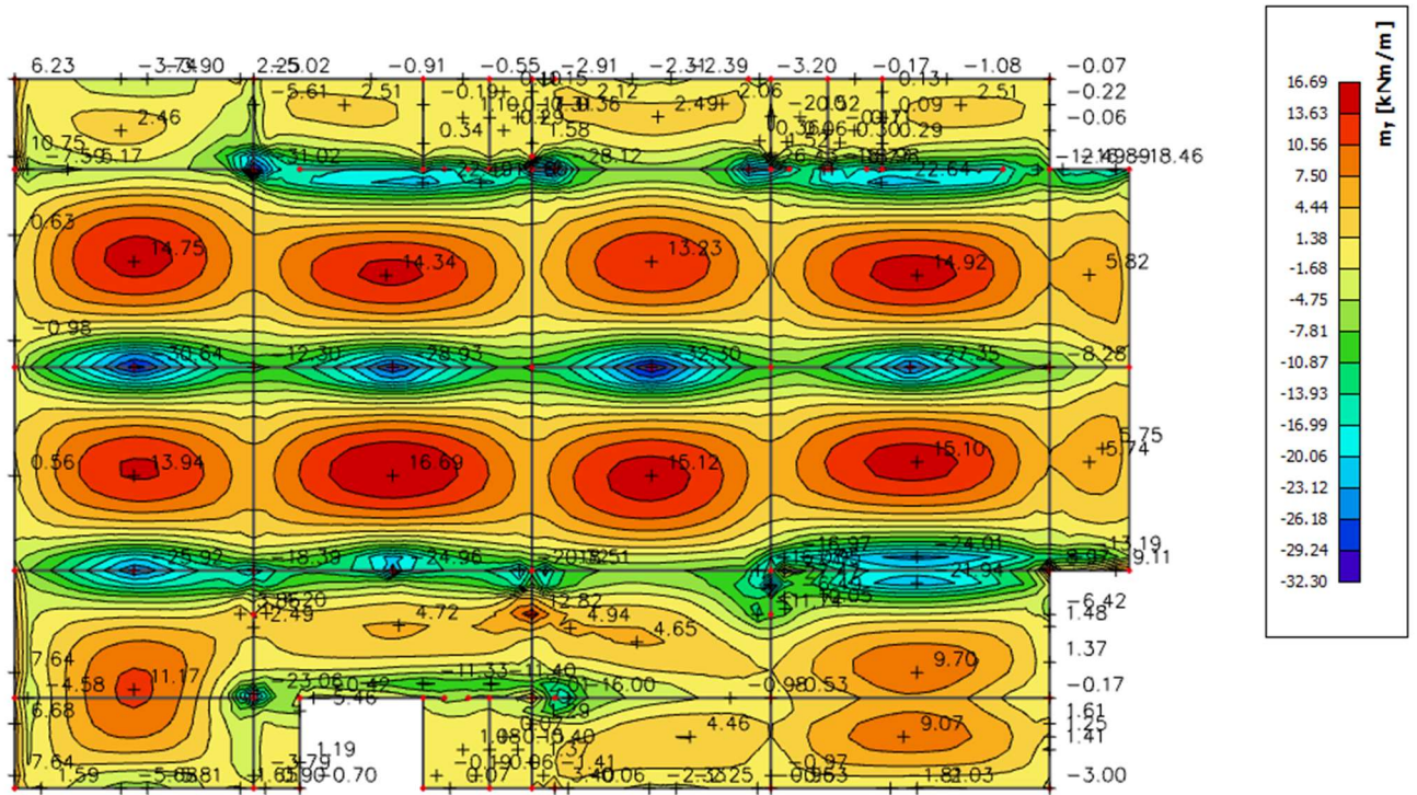
Slika 6.15 Moment savijanja M_{Ed,y} ( \text{kNm/m} ) za GSN-1
