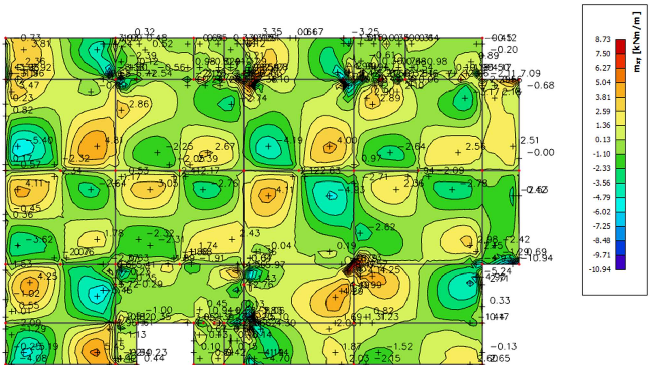
Slika 6.16 Moment savijanja M_{Ed,xy} ( \text{kNm/m} ) za GSN-1
