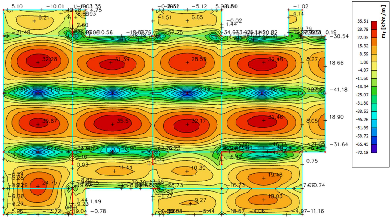
Slika 6.3 Moment savijanja M_{Ed,y} ( \text{kNm/m} ) za GSN-1
