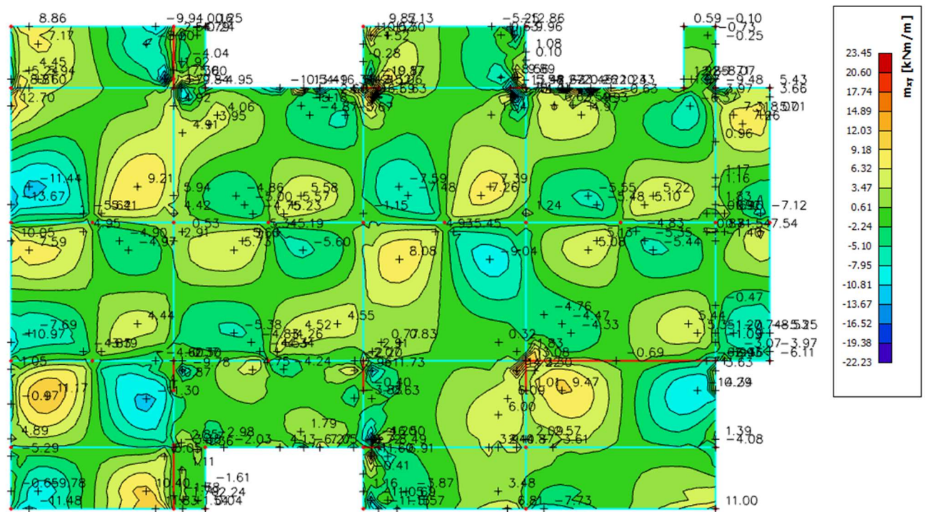
Slika 6.4 Moment savijanja M_{Ed,xy} ( \text{kNm/m} ) za GSN-1
