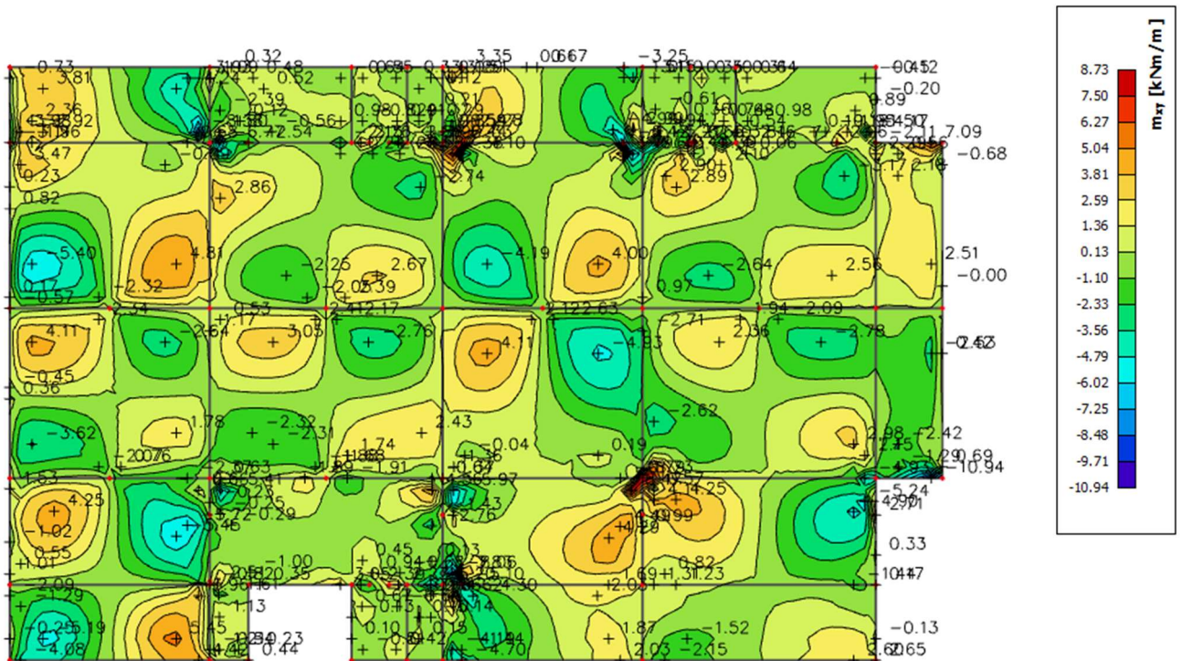
Slika 6.16 Moment savijanja M_{Ed,xy} ( \text{kNm/m} ) za GSN-1
