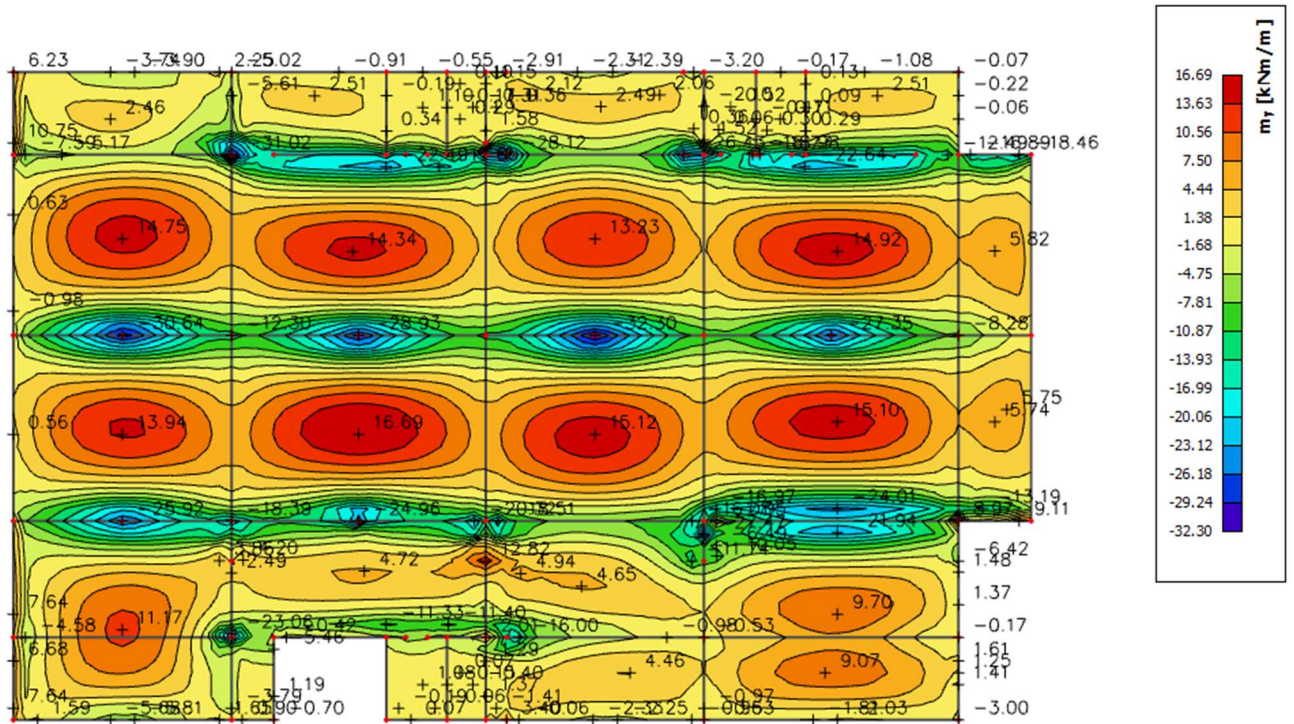
Slika 6.15 Moment savijanja M_{Ed,y} ( \text{kNm/m} ) za GSN-1
