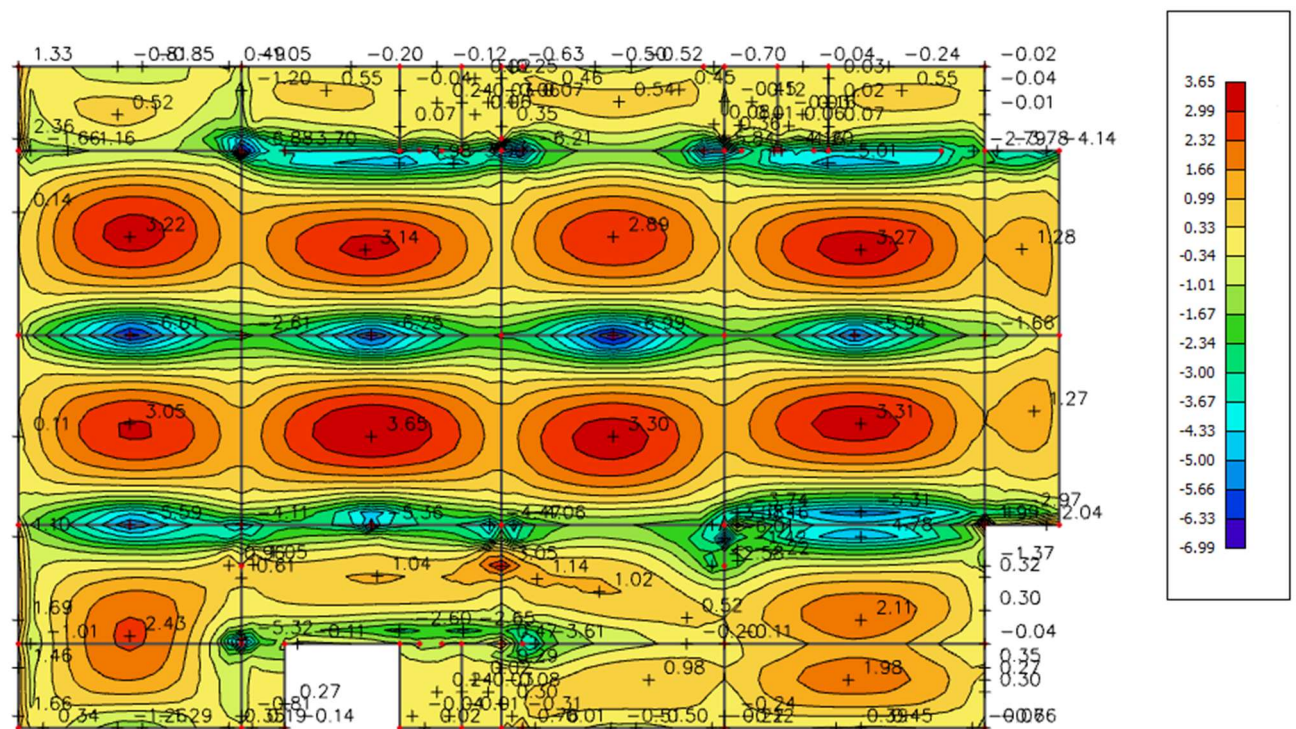
Slika 6.20 Potrebna površina armature A_s(\text{cm}^2/\text{m}) u y smjeru
