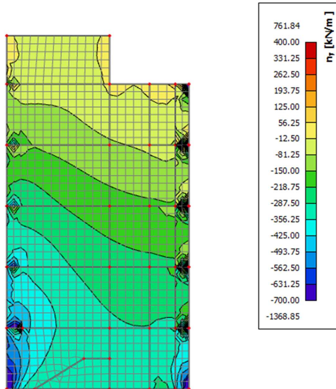
Slika 8.6 Uzdužne sile n_{Ed} [ \text{kN/m} ] u smjeru Y, u zidovima za anvelopu GSN
