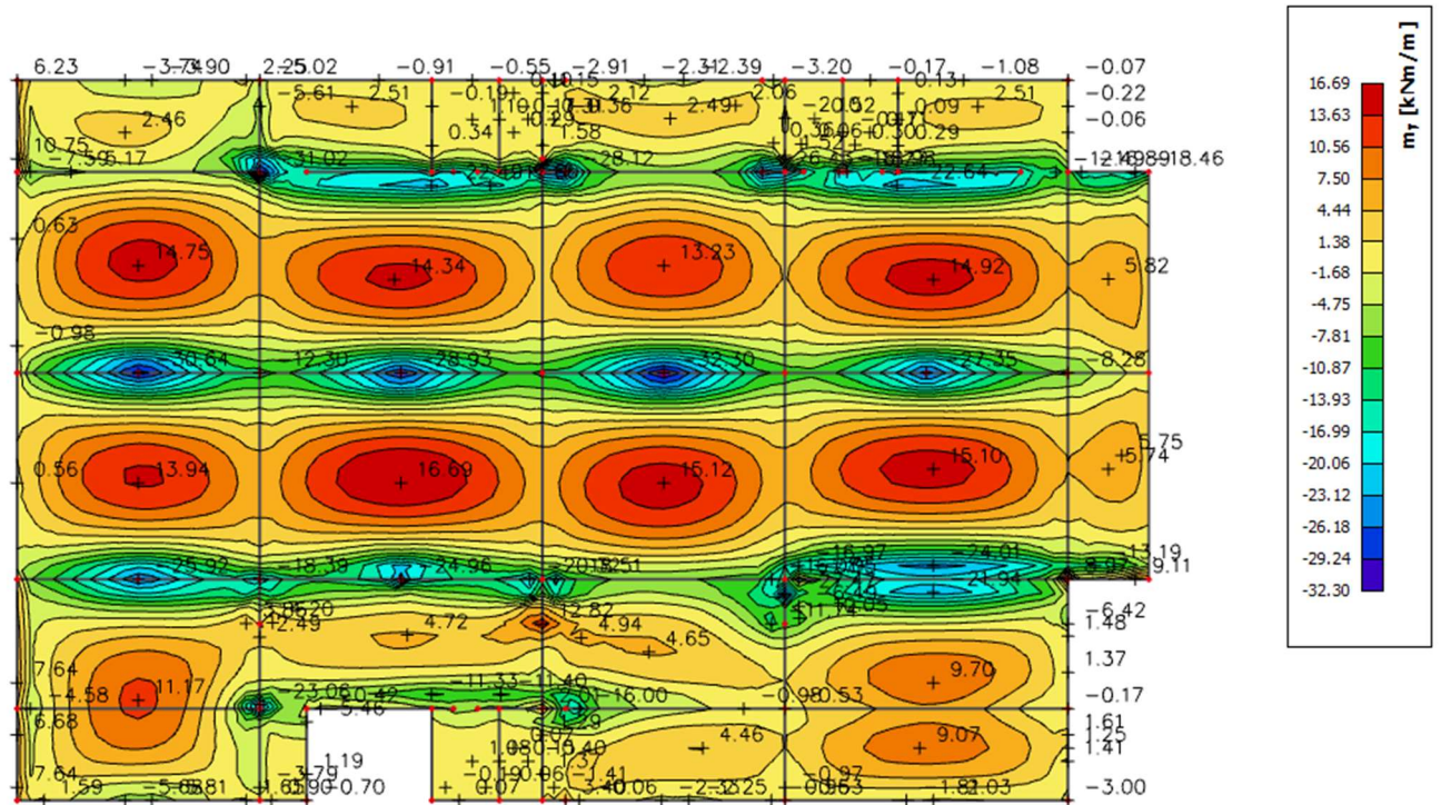
Slika 6.15 Moment savijanja M_{Ed,y} (kNm/m) za GSN-1
