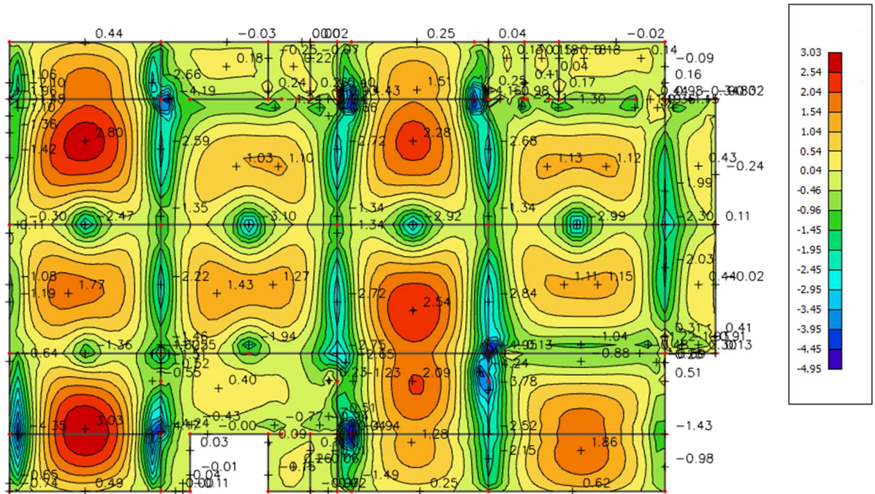
Slika 6.19 Potrebna površina armature A_s(\text{cm}^2/\text{m}) u x smjeru
