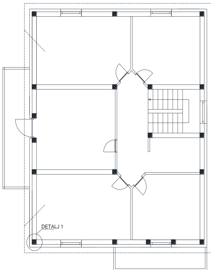
DETALJ 1
