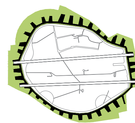
*4. Obrnuti blok
