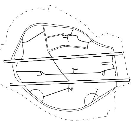
*1. Prazno polje
