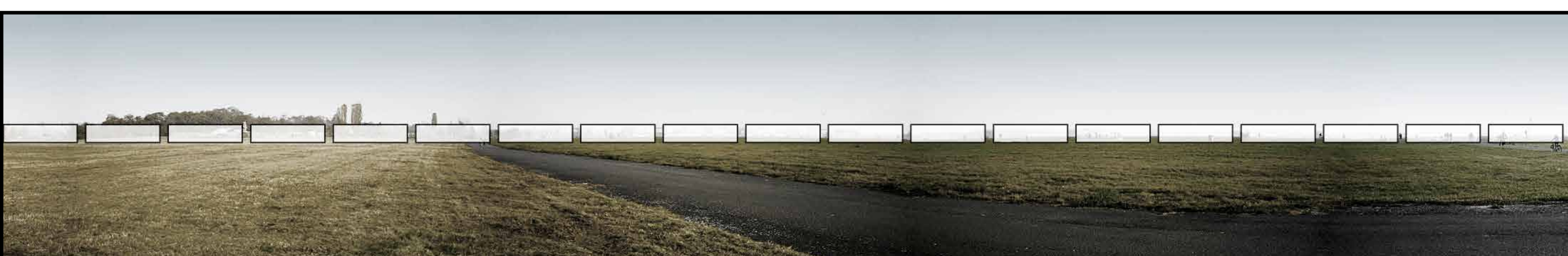
*1. Prazno polje
