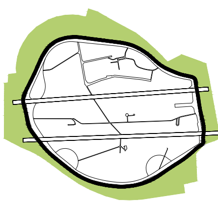
*2. Definiiranje ruba
