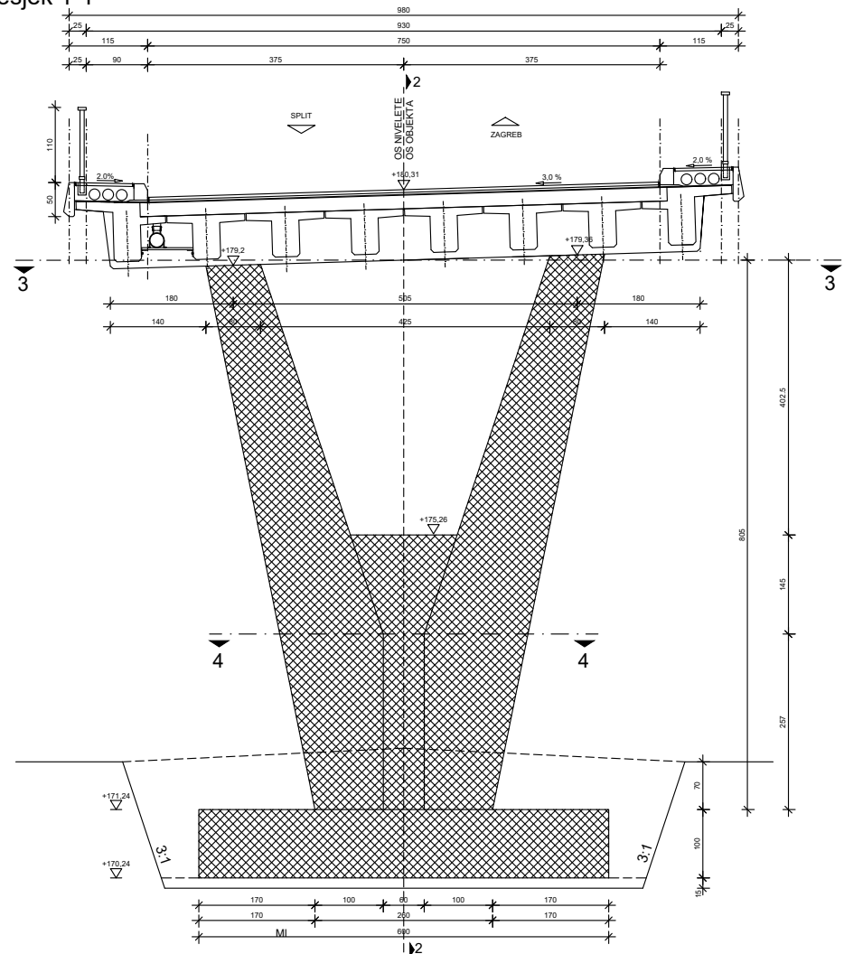
Presjek 1-1
