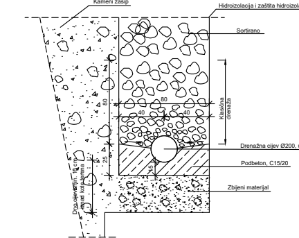
Detalj drenage
