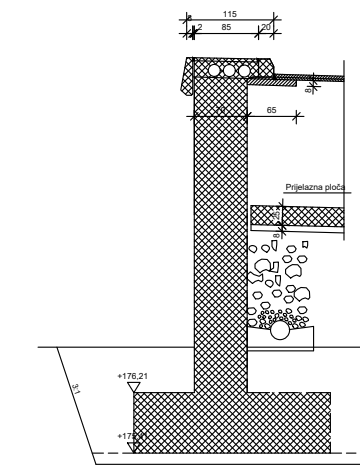
Presjek 7-7
