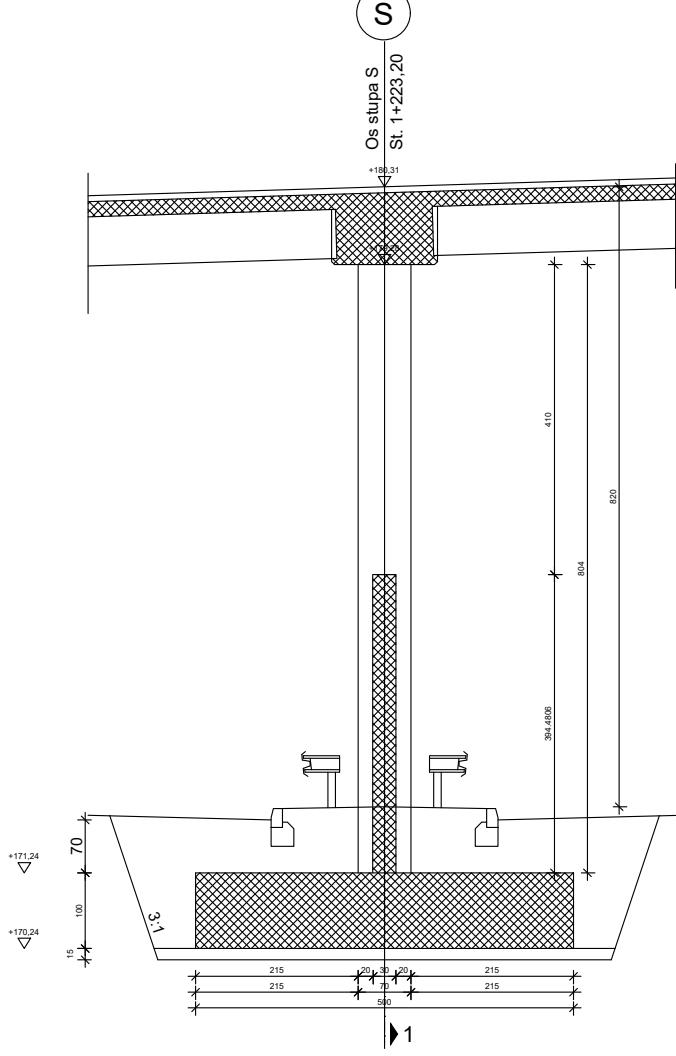
Presjek 2-2
