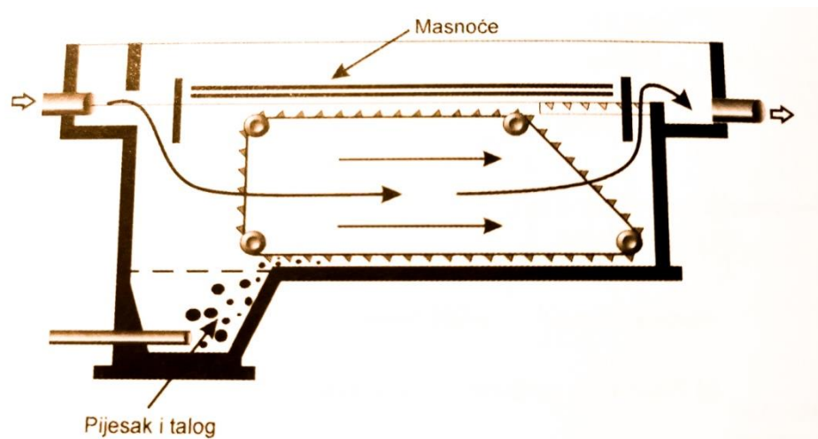
Slika 4.6 Bazen- taložnik i mastolov
