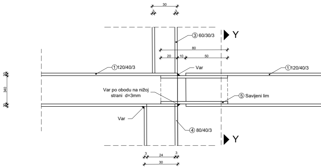
Detalj D 2 1:2
