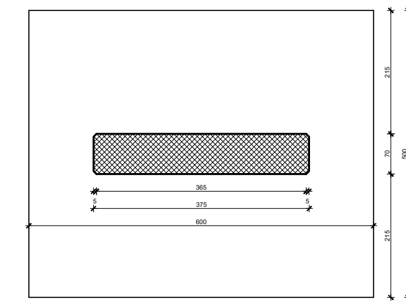
Presjek 4-4
