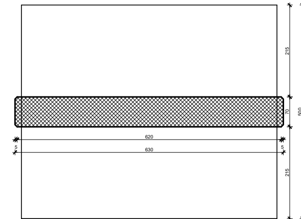
Presjek 4-4
