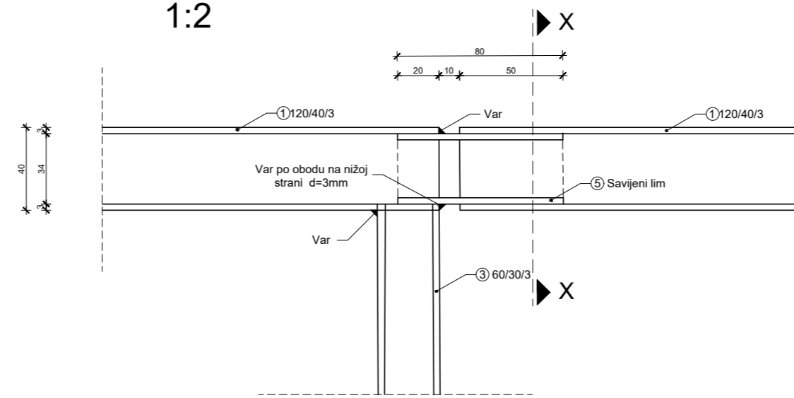
Detalj D 2 1:2
