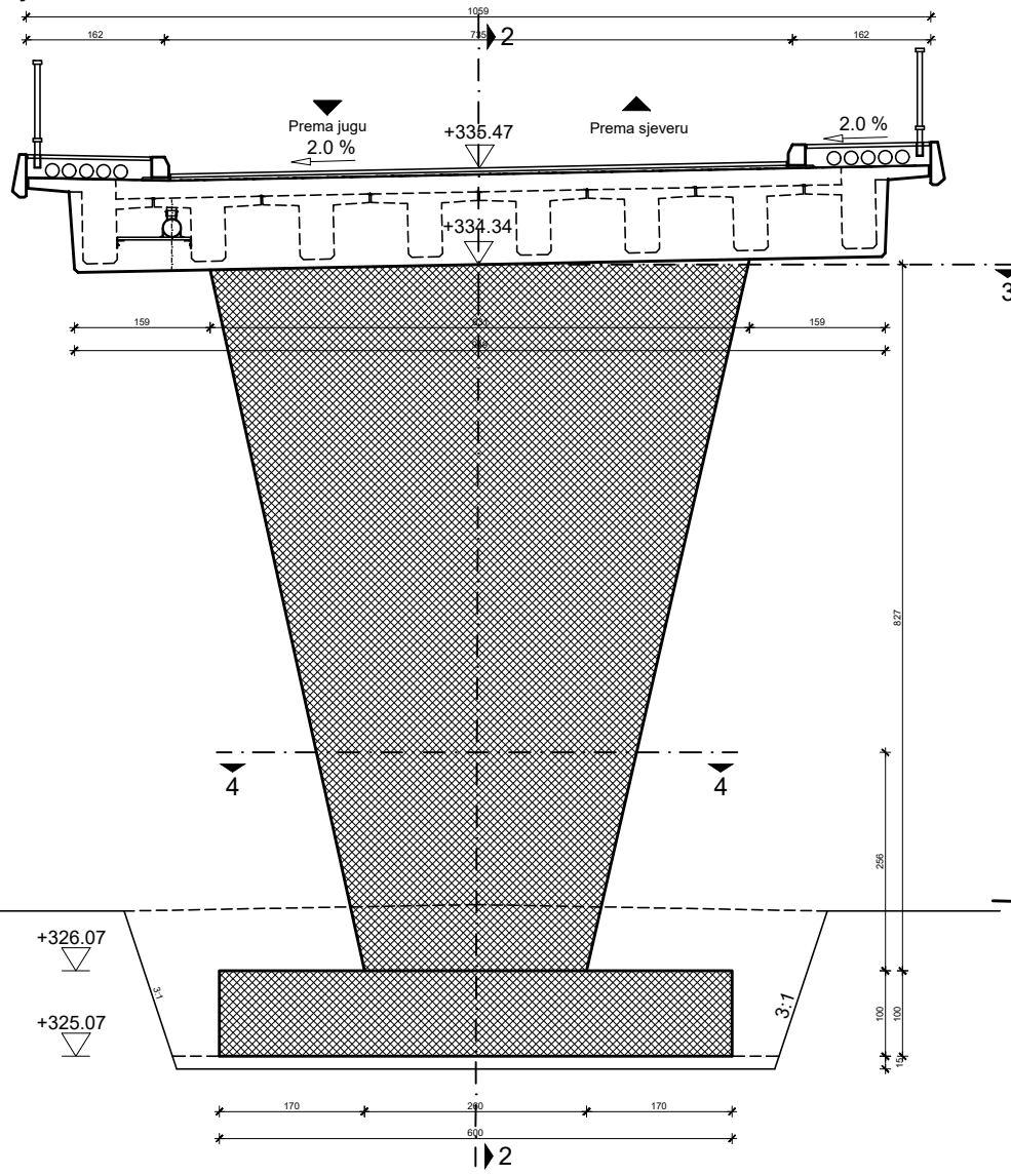
Presjek 1-1
