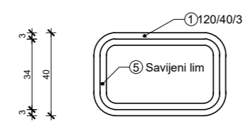
PRESJEK X-X
