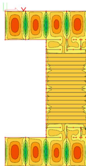
Slika 6.1.2 Moment savijanja M_{Ed,x} (kNm/m) za GSN-1
