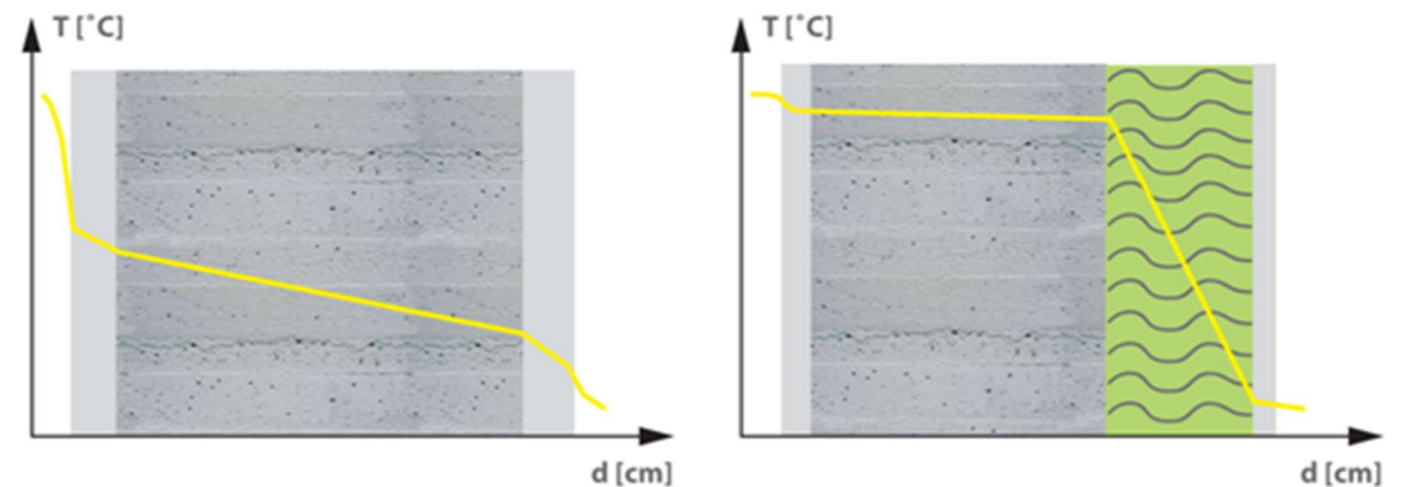
Temperaturne krivulje za neizolirani i izolirani AB zid ( Tl s vanjske strane), izvor: EIHP
