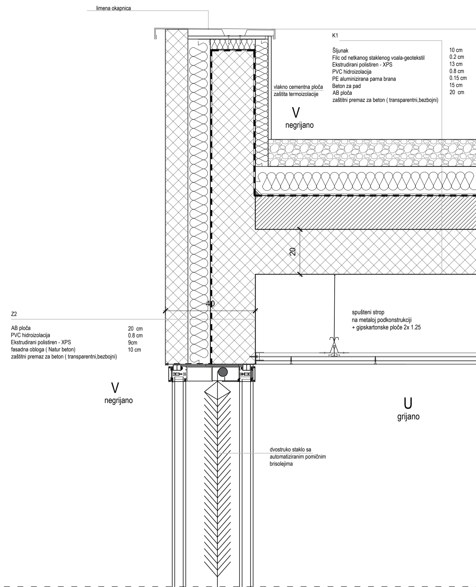
D3 DETALJ NEPROHODNOG KROVA
