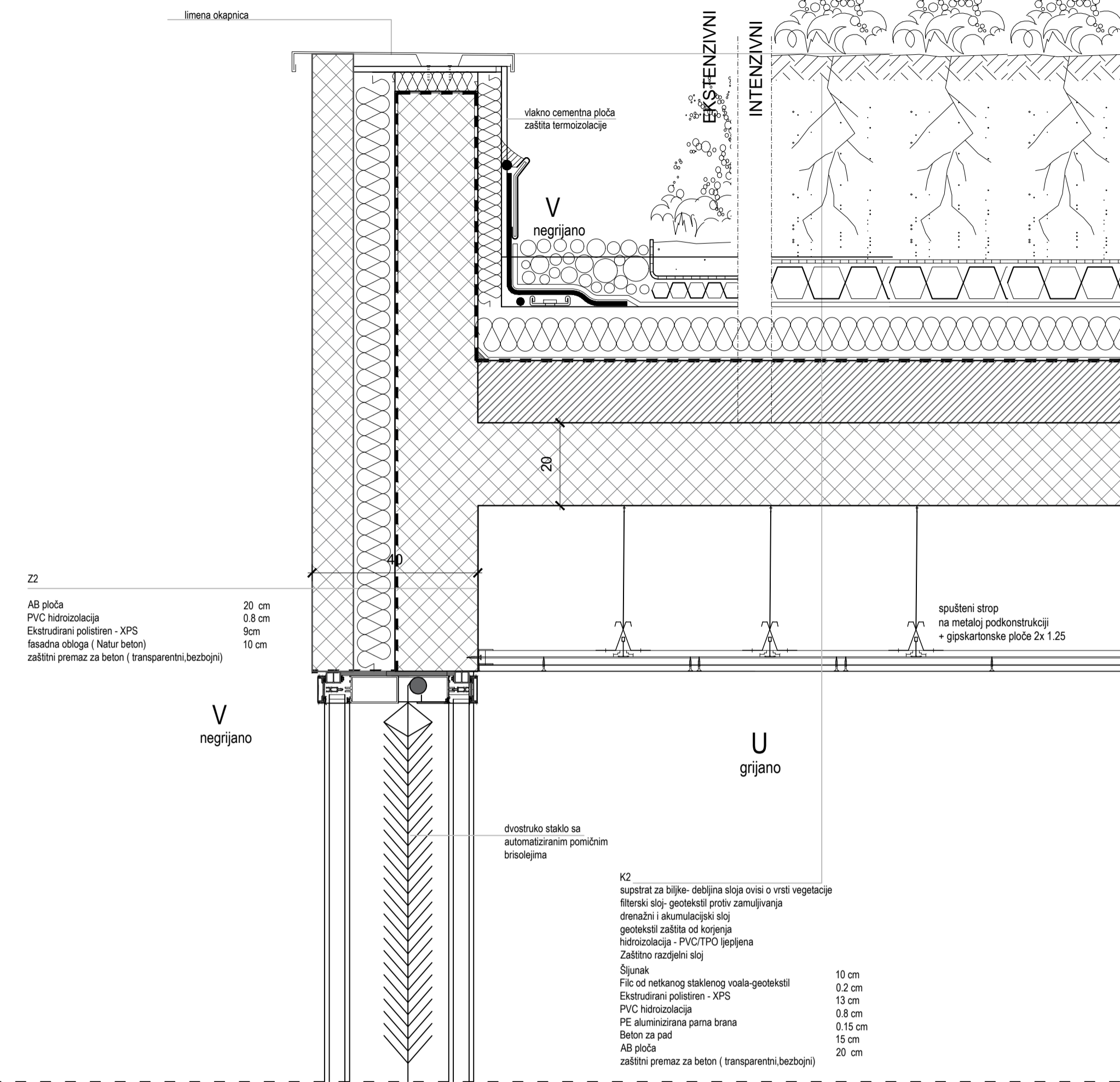
D4 DETALJ ZELENOG KROVA
