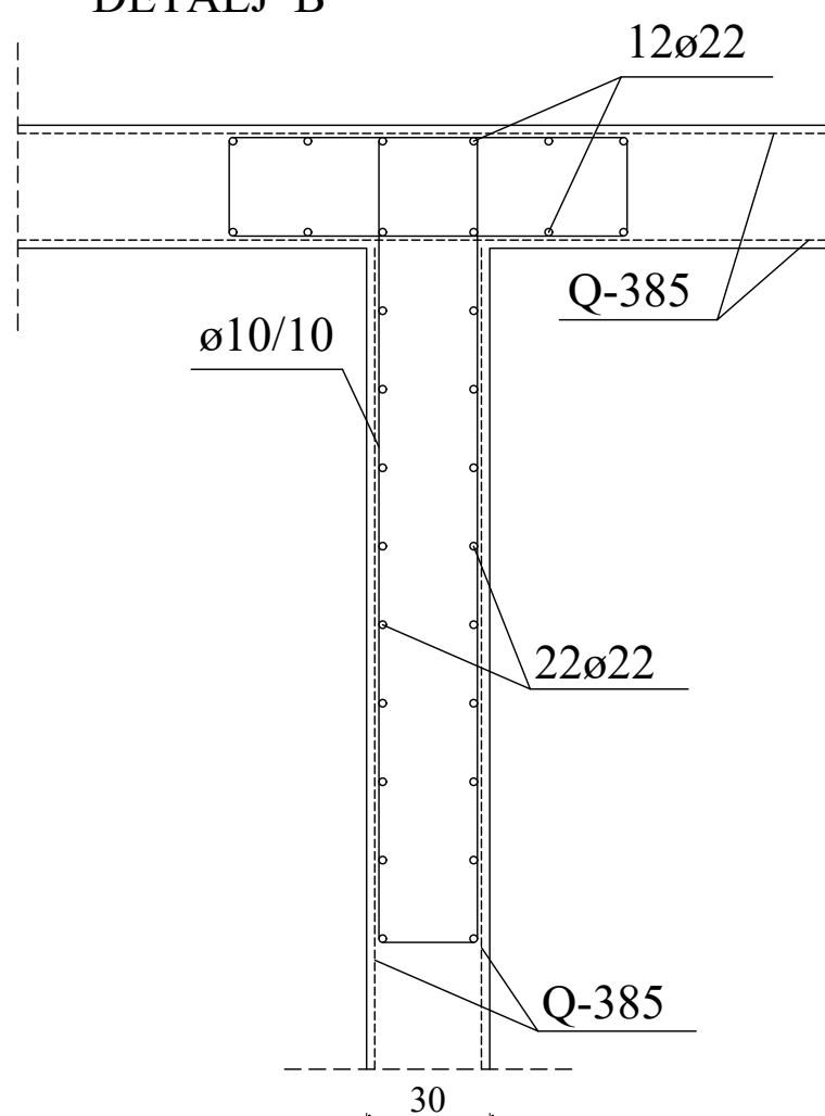
DETALJ B
