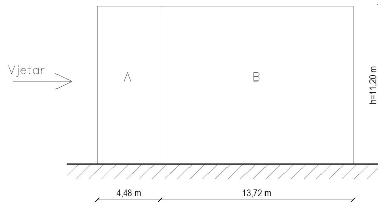
Slika 8.16. Vjetrovne zone za smjer y
