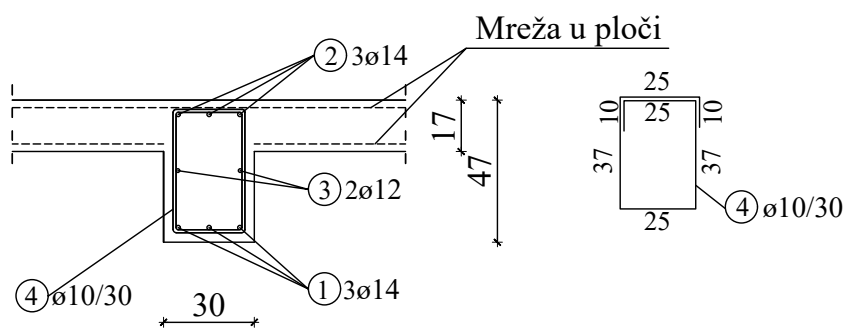
PRESJEK 2-2
