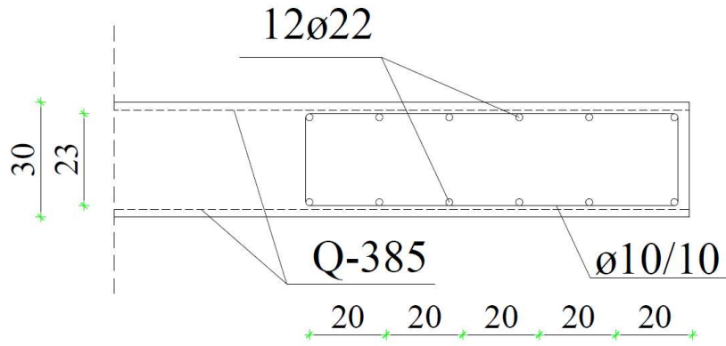
Slika 13.9. Prikaz armature karakterističnog zida
