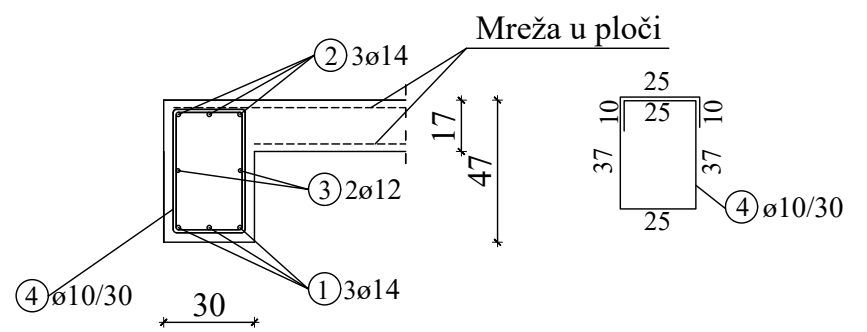
PRESJEK 2-2
