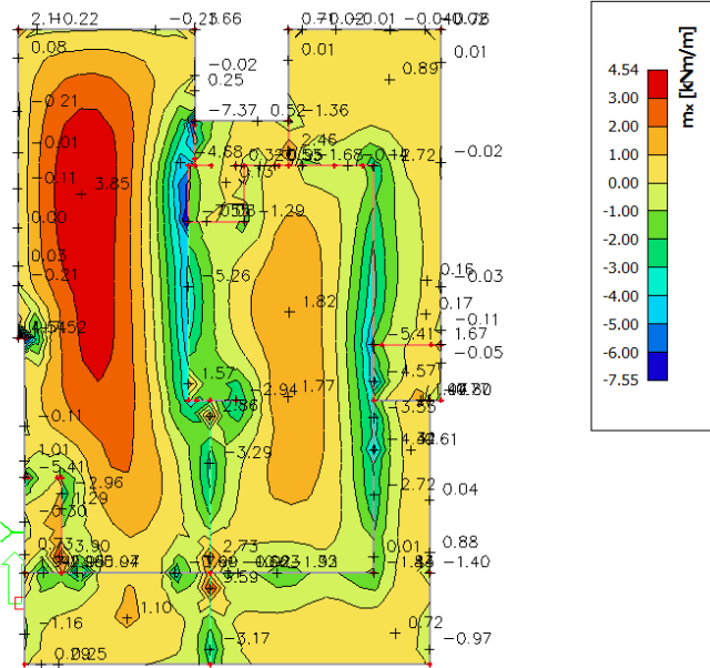
Slika 43. Moment savijanja M_x
