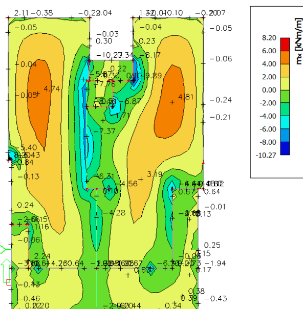
Slika 30. Moment savijanja M_x
