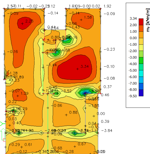
Slika 31. Moment savijanja M_y
