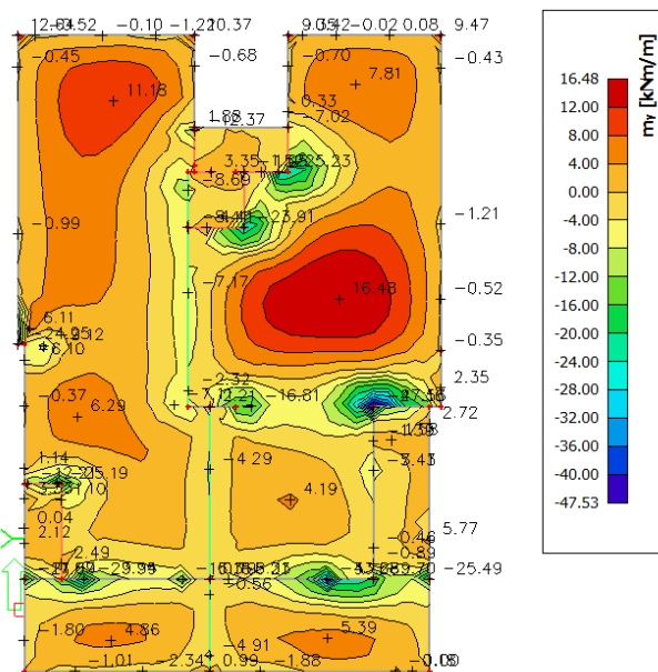
Slika 35. Moment savijanja M_y
